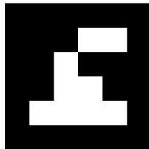
♟ BP6 ID: 29
