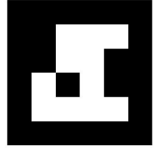
♝ BR2 ID: 19
