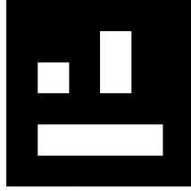
♟ WP6 ID: 13
