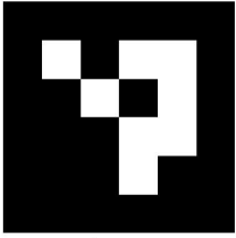
♔ WK ID: 0
