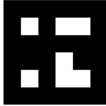
♟ BB2 ID: 21
