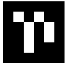
♞ BP4 ID: 27
