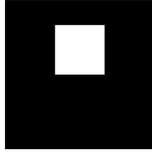
♛ BQ ID: 17
