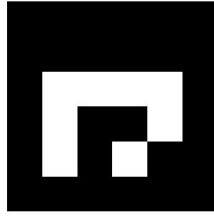
♑ WQ ID: 1
