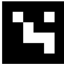
♞ BP2 ID: 25
