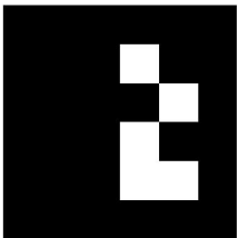
♞ BP5 ID: 28
