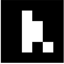
♚ BK ID: 16
