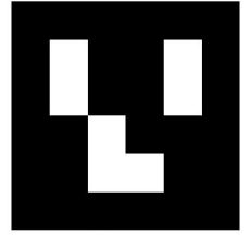
♗ WR2 ID: 3
