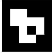
♜ WP2 ID: 9
