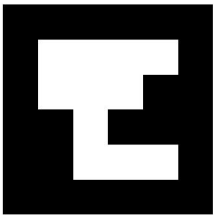
♟ BP1 ID: 24
