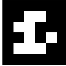
♜ BR1 ID: 18
