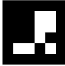
♖ WR1 ID: 2
