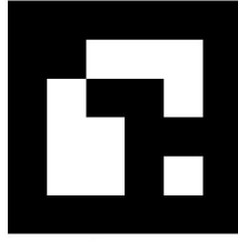
♙ WB2 ID: 5
