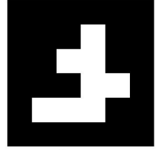
♟ WP8 ID: 15
