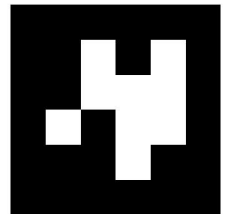
♟ BP8 ID: 31
