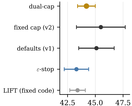
Dream-7B + s1K
