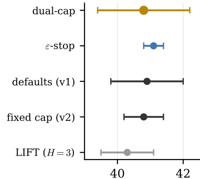
LLaDA-1.5 + s1K
