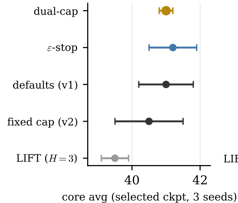
LLaDA-8B + s1K
