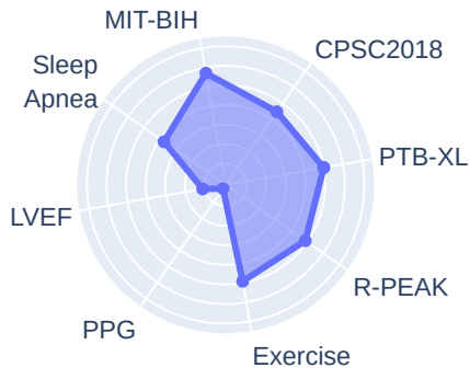
ST-MEM
