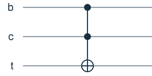
AND2 / Toffoli
