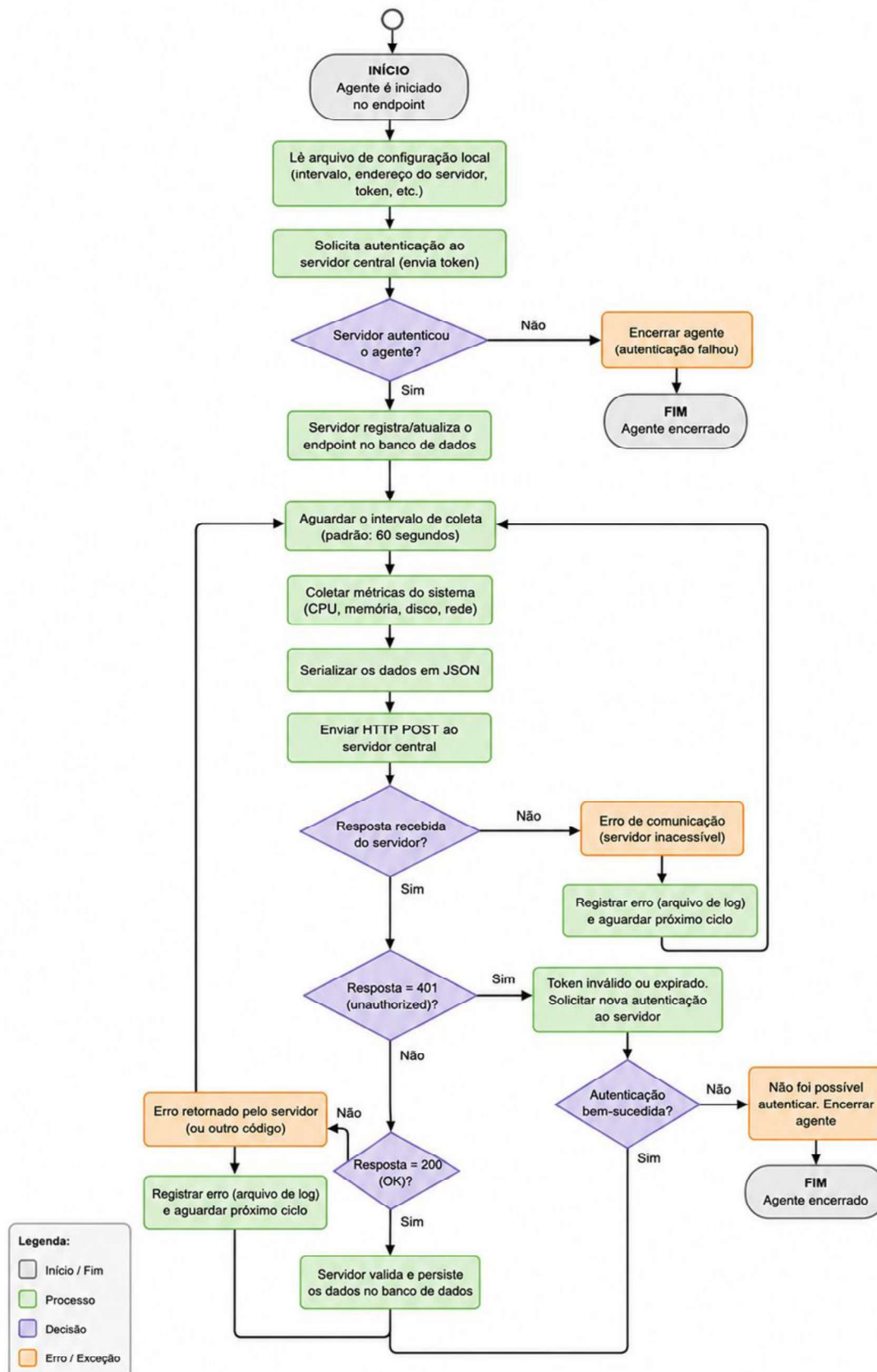
Figura 02: Fluxo de coleta e envio de métricas.
