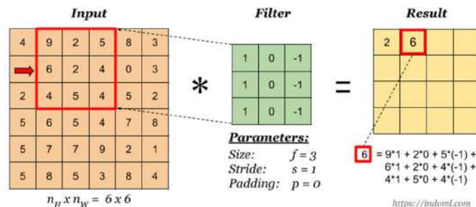
Gambar 2.6 Operasi Konvolusi
