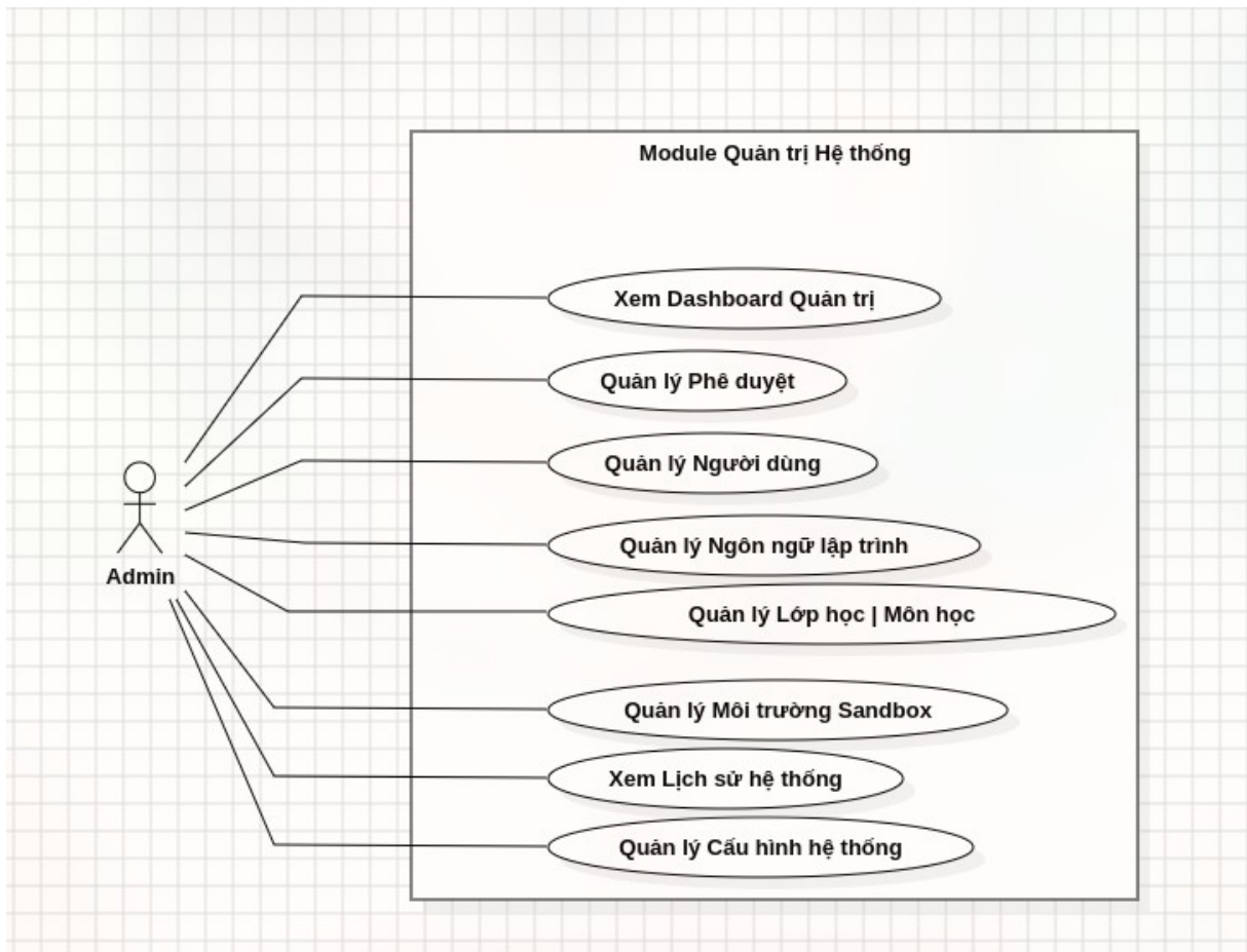
Hình 2.4. Biểu đồ Use Case Module Quản trị Hệ thống
