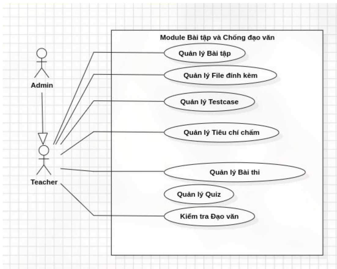
Hình 2.6. Biểu đồ Use Case Module Bài tập và Chống đạo văn
