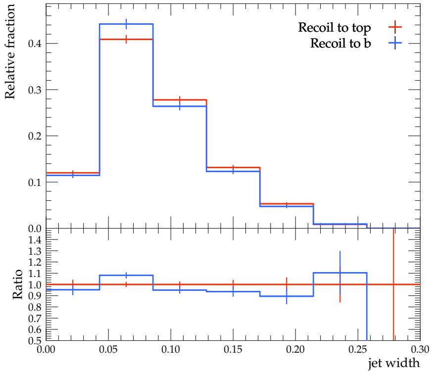
Bar chart of C-jet width
