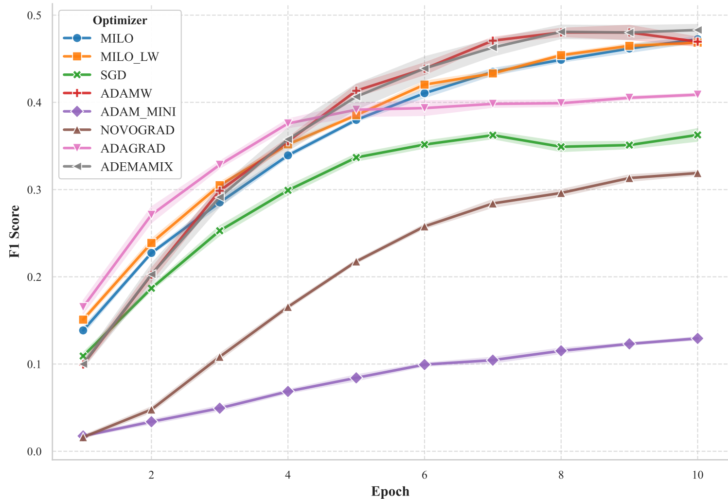
Validation F1 Score for RESNET34_CIFAR100 Experiment
