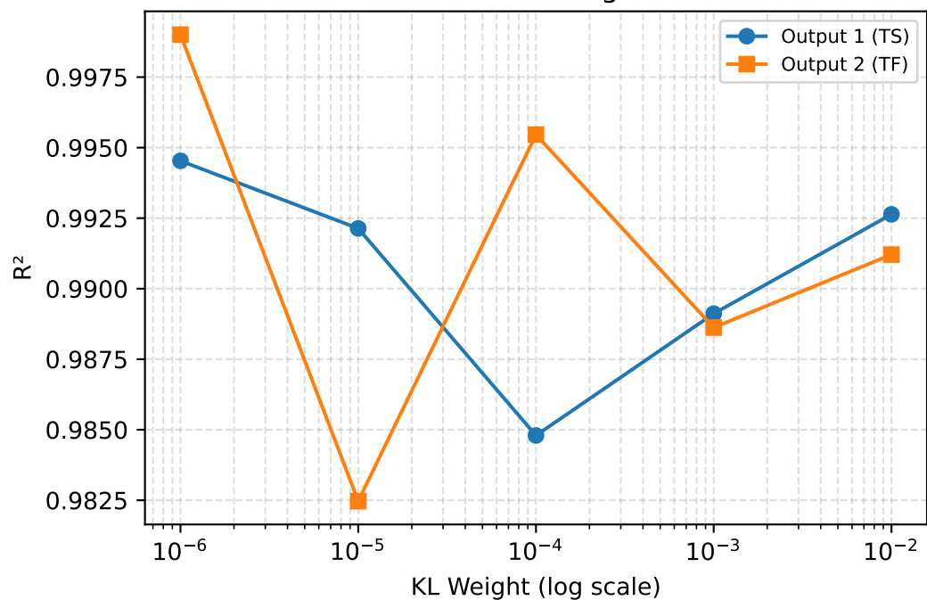
R 2 vs KL Weight
