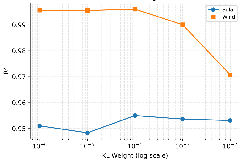
R 2 vs KL Weight
