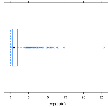
(d) Boxplot
