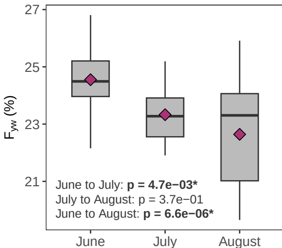
Prior: 0.2/0.8
