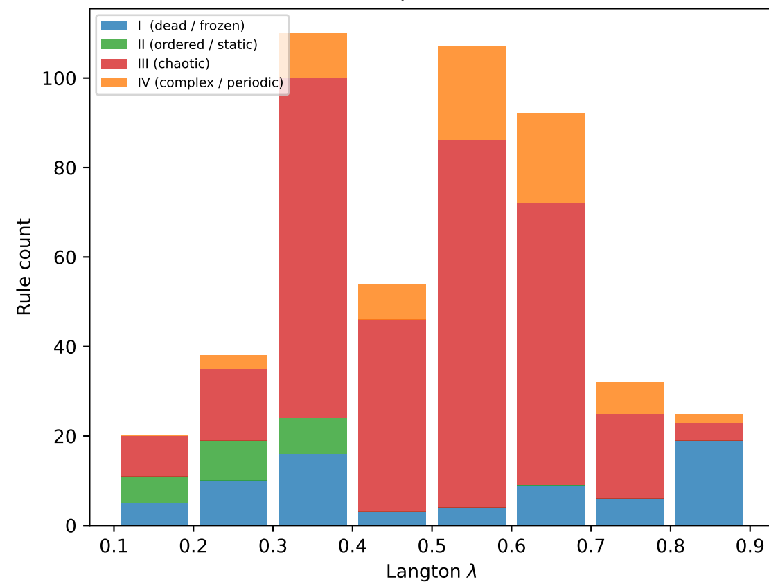
(d) Phase prevalence vs \lambda
