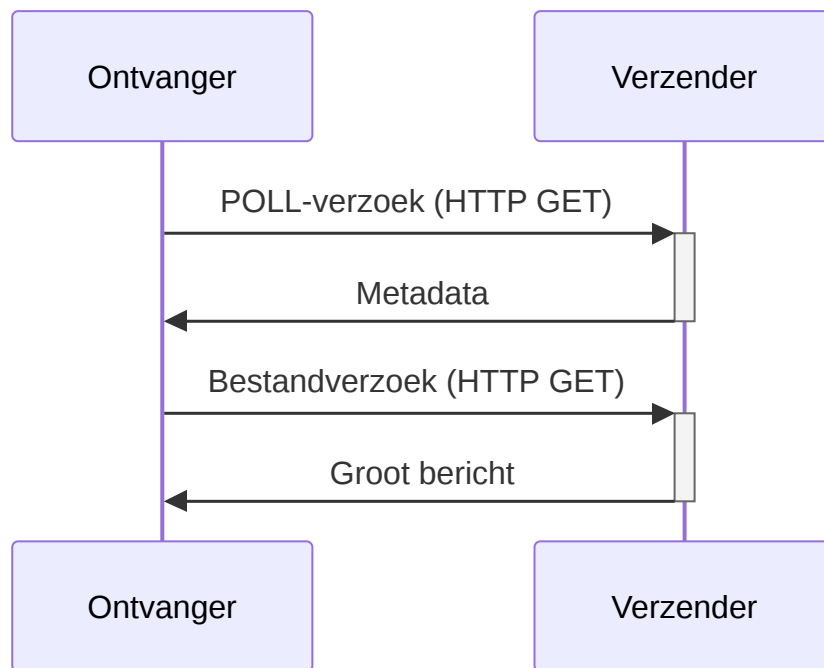
Figuur 4 Uitwisseling groot bestand via Grote Berichten file service van de verzender
