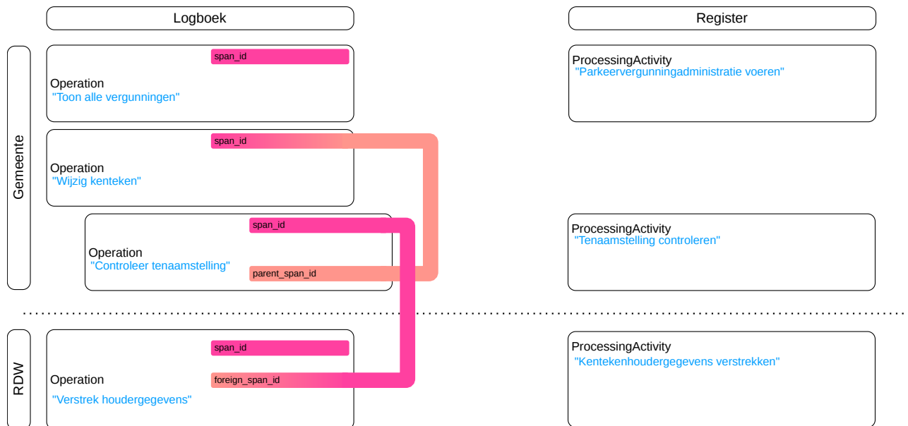
Figuur 17 Afbeelding voorbeeld span_id, parent_span_id en foreign_span_id bij Gemeente en RDW
