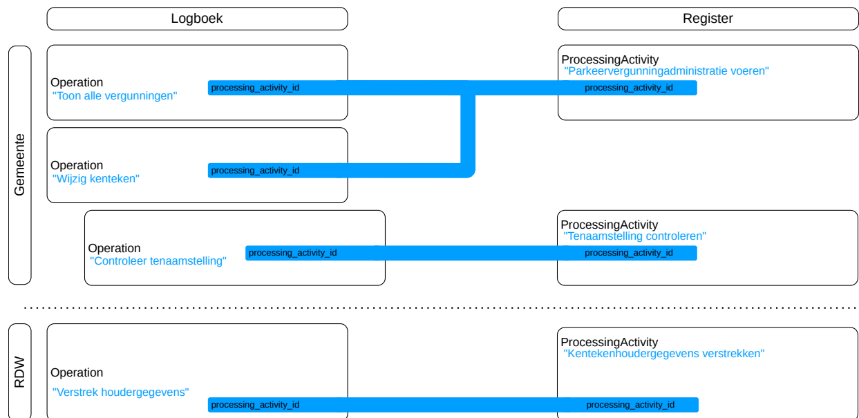
Figuur 15 Afbeelding voorbeeld processing_activity_id en parent_processing_activity_id bij Gemeente en RDW
