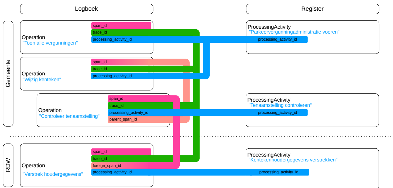
Figuur 18 Afbeelding Voorbeeld met alle span, trace en processing elementen
