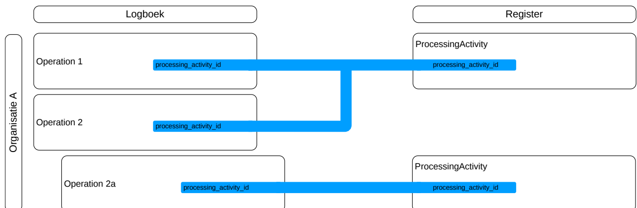
Figuur 7 Afbeelding relaties processing_activity_id tussen Logboek en Register met parent_processing_activity_id
