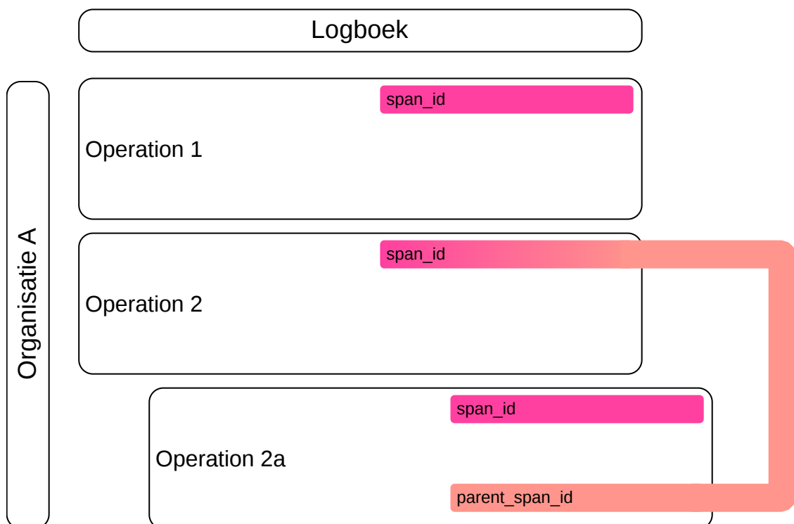
Figuur 13 Afbeelding span_id en parent_span_id
