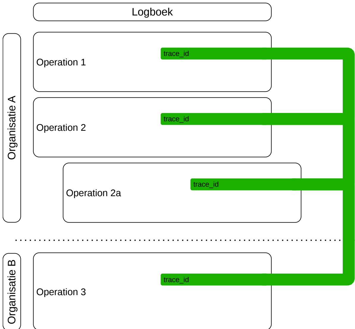
Figuur 11 Afbeelding relaties trace_id en meerdere organisaties
