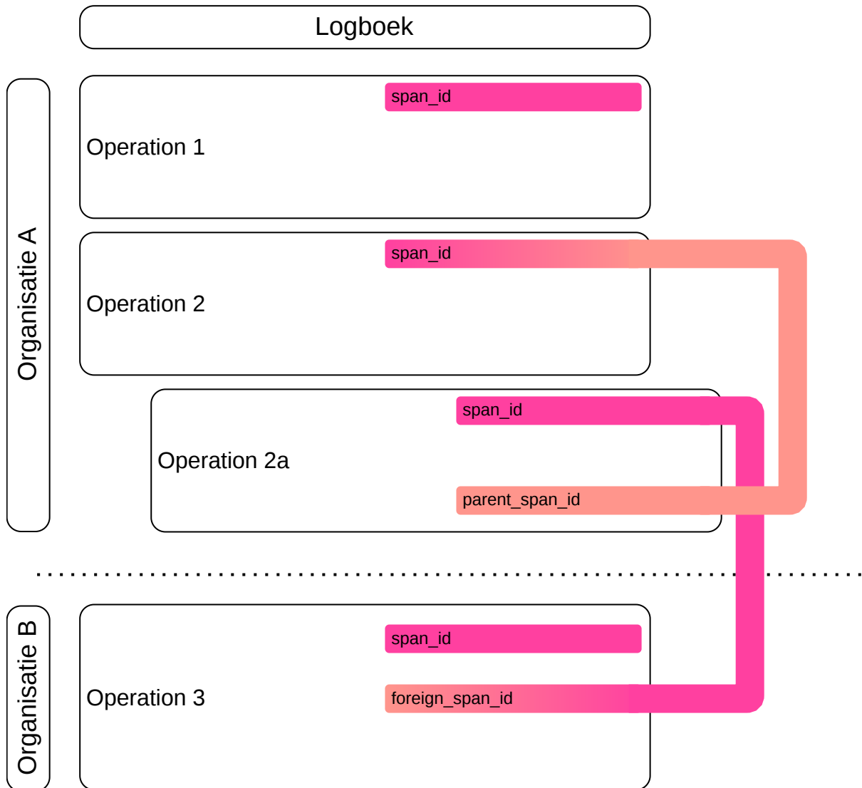
Figuur 13 Afbeelding span_id , parent_span_id en foreign_span_id
