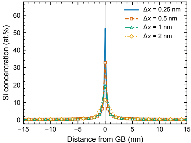
Set 20261001/1, Si, Dirichlet GB BC
