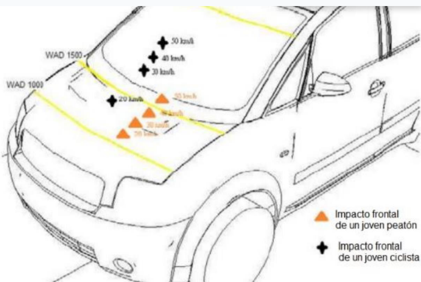
Diagrama técnico forense con puntos de impacto sobre vehículo genérico para peatón joven y ciclista joven a distintas velocidades (20-50 km/h), con referencias WAD.
