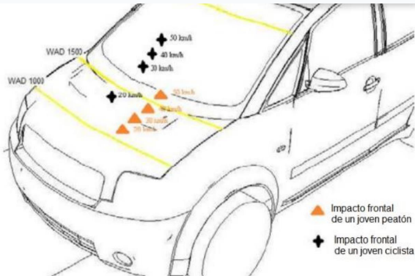
Diagrama técnico forense con puntos de impacto de peatón y ciclista sobre capó y parabrisas según velocidad, con referencias WAD 1000 y WAD 1500.
