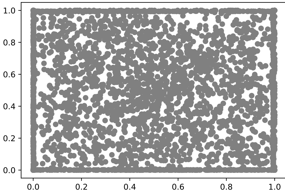
Nuages projeté dans les dimension 0 et 1
