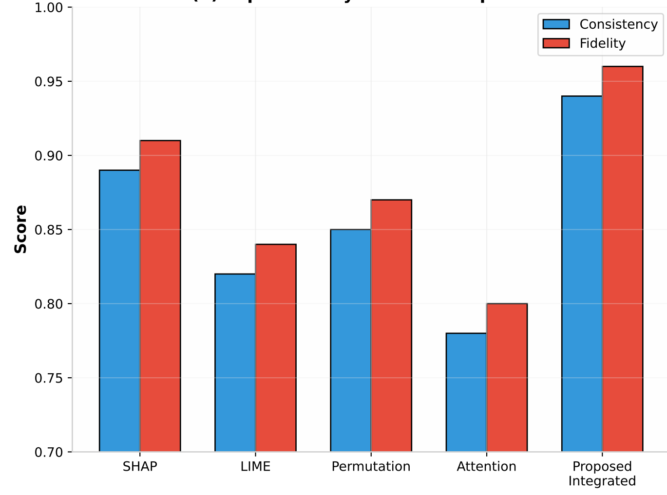
(d) Explainability Method Comparison
