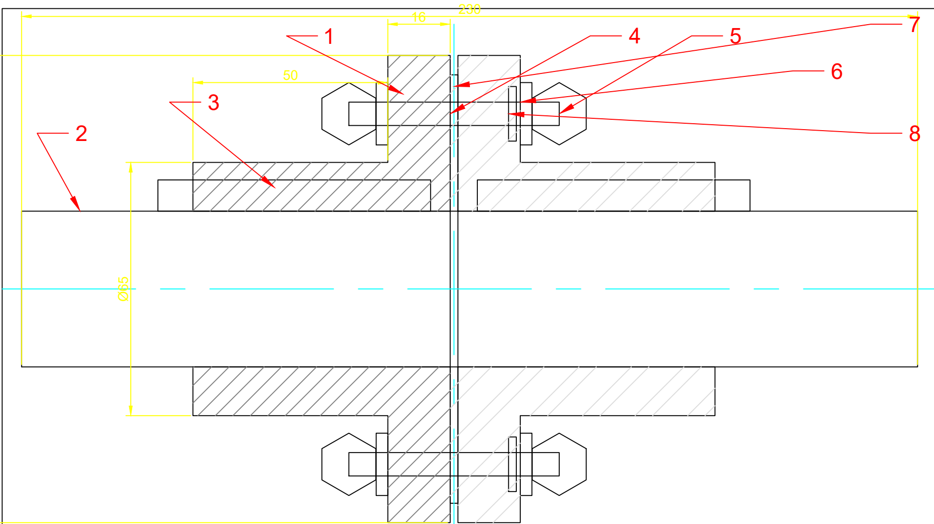
LONGITUDINAL HALF-SECTION A-A
