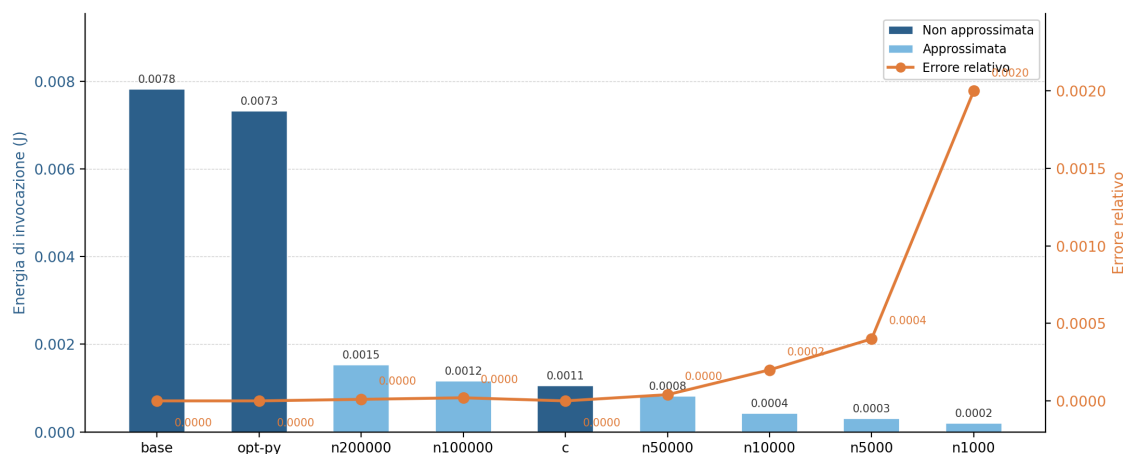
Figura 5.1: Energia di invocazione ed errore relativo delle varianti di PiLeibniz. Le varianti esatte presentano errore nullo, mentre le varianti approssimate riducono progressivamente l'energia diminuendo il numero di termini della serie. L'errore resta contenuto per le varianti intermedie e cresce solo per le approssimazioni più spinte, evidenziando una frontiera energia-accuratezza densa e modulabile.
