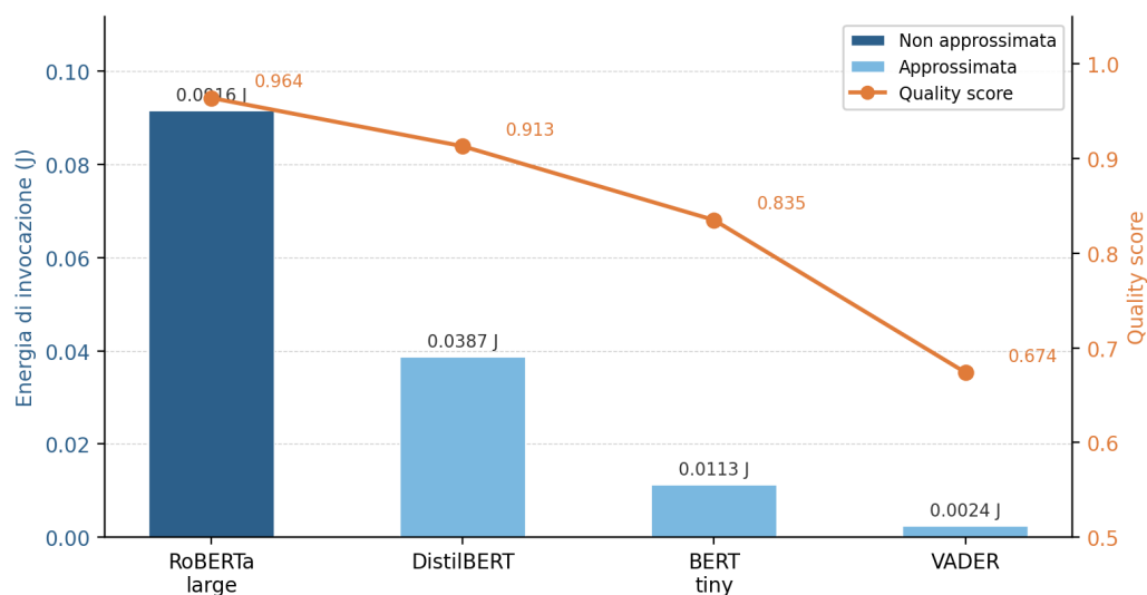
Figura 5.2: Energia di invocazione e quality_score delle varianti di SentimentAnalysis. Il passaggio a modelli più leggeri riduce sensibilmente il costo energetico, ma la qualità diminuisce per salti discreti, riflettendo la natura architetturalmente distinta delle varianti ML.
