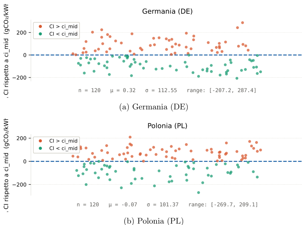
Figura 5.11: Distribuzione annuale della carbon intensity per zona e fasce utilizzate per il campionamento dei timestamp dell'Esperimento 2. La selezione bilanciata tra valori bassi, medi e alti evita che il campione sia concentrato solo attorno alle condizioni più frequenti della rete.
