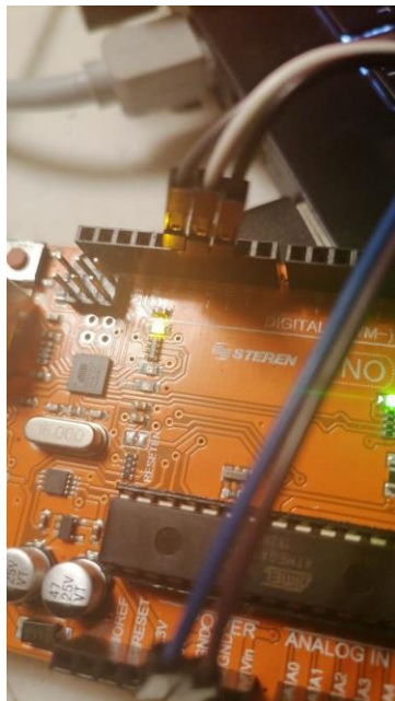
Imagen 1.2 Conexión a Arduino, Pines 10,11 y 12. DIN pin 12, CS pin 10 y CLK pin 11.
