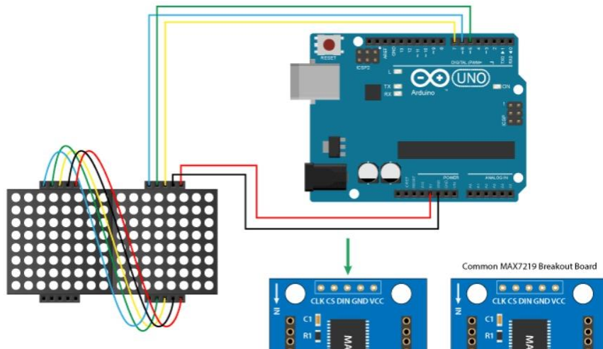
Imagen 1.1 Conexión de pines Arduino a matriz led principal.
