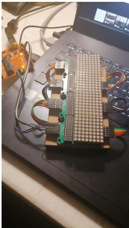
Imagen 1.3 Conexión en cascada de matrices led
