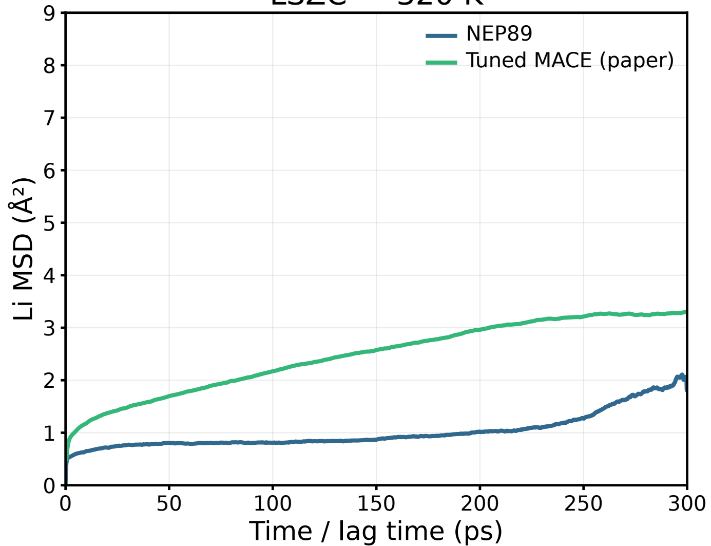
LSZC — 320 K
