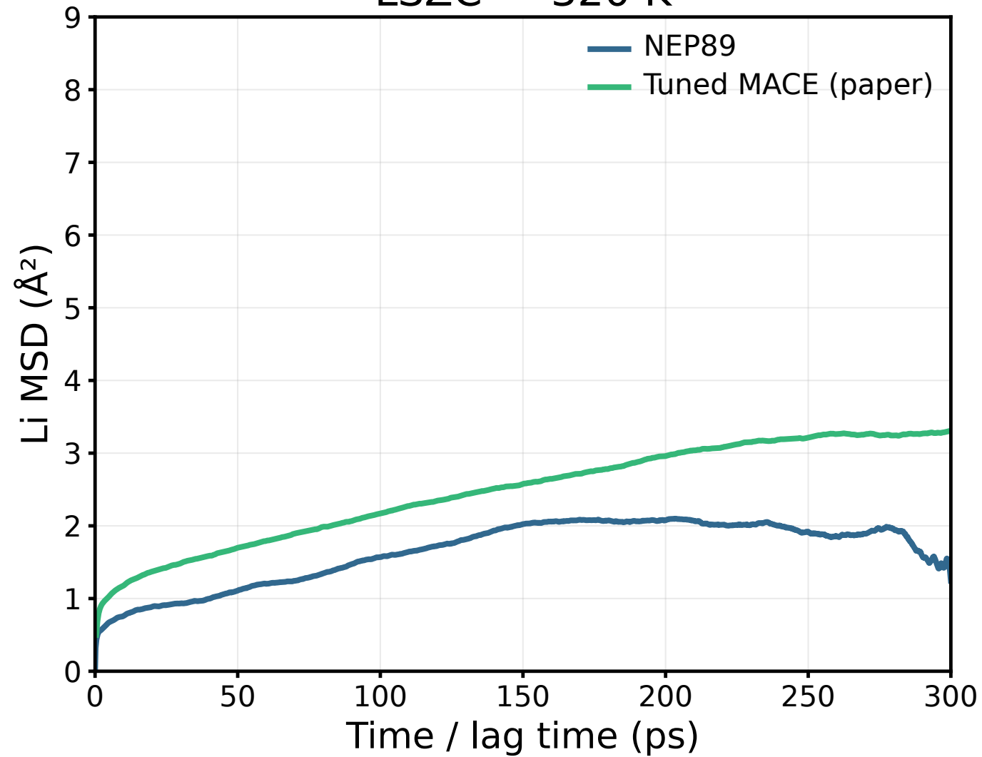
LSZC — 320 K
