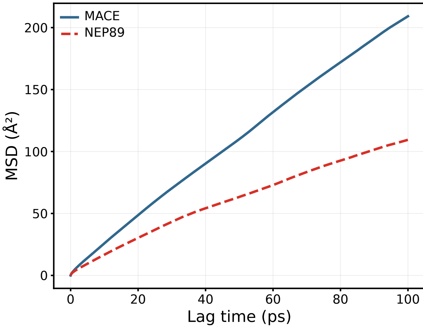
700 K: Li MSD
