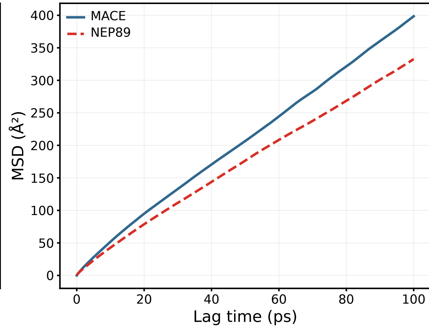
900 K: Li MSD
