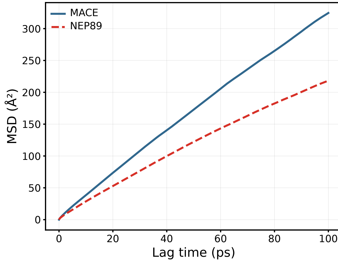
800 K: Li MSD
