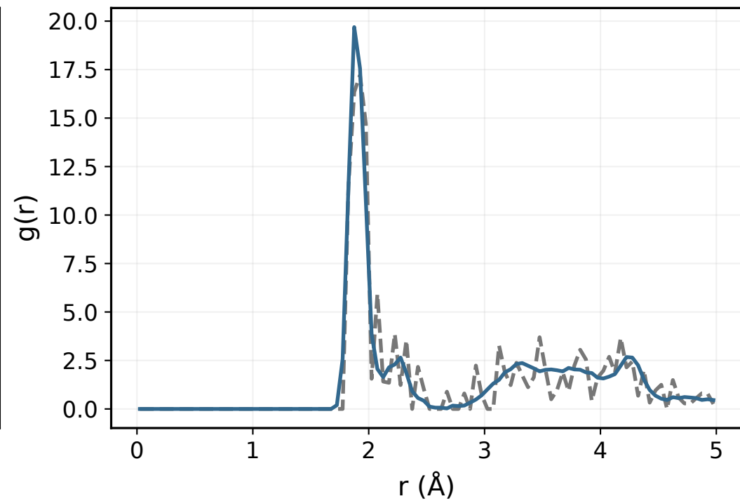
Li-Cl
