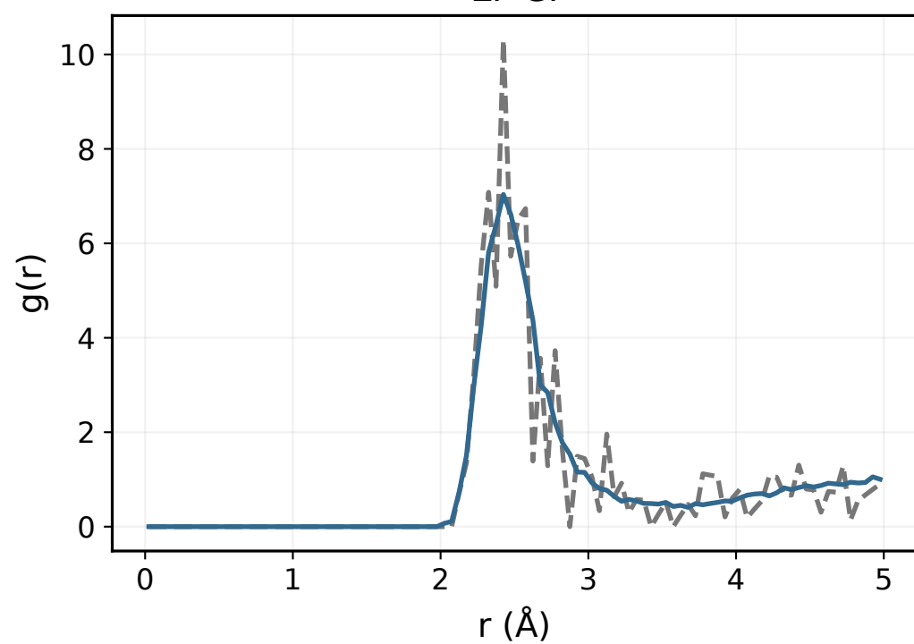
Li-Cl
