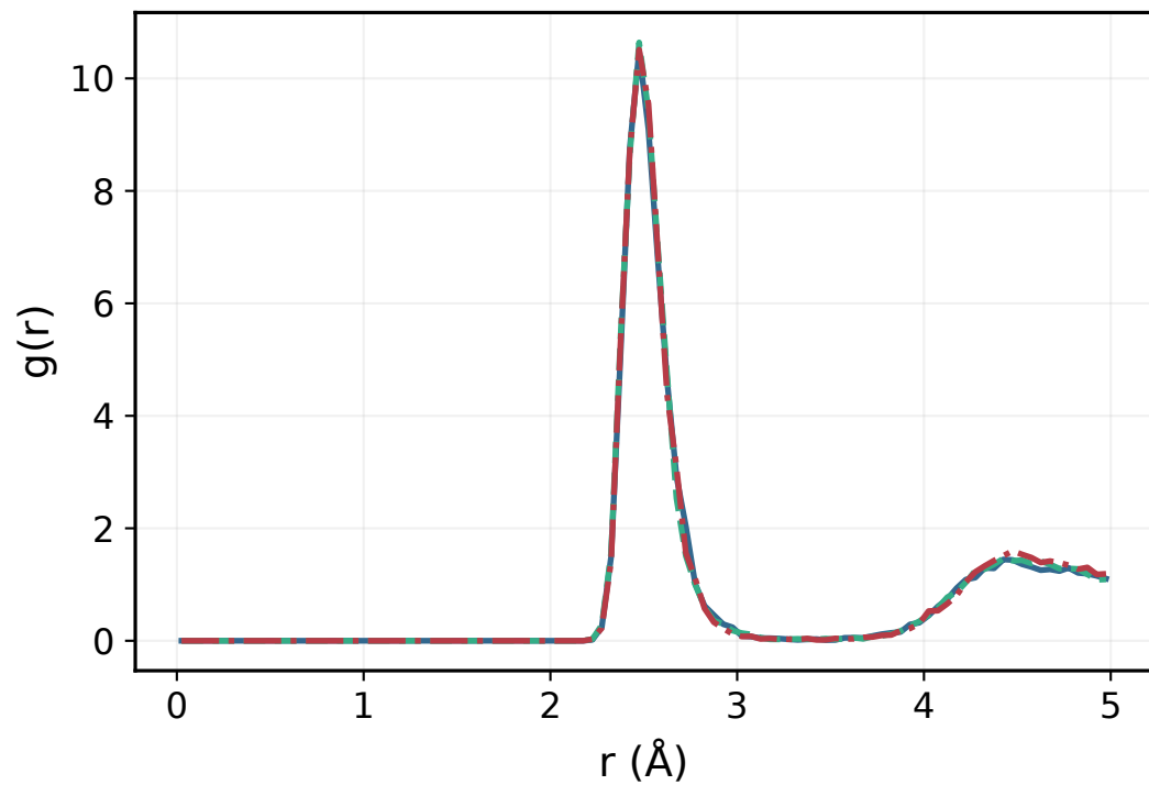
Cl-Cl
