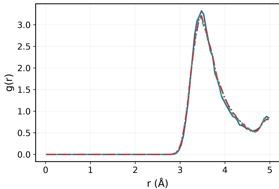
Cl-Cl
