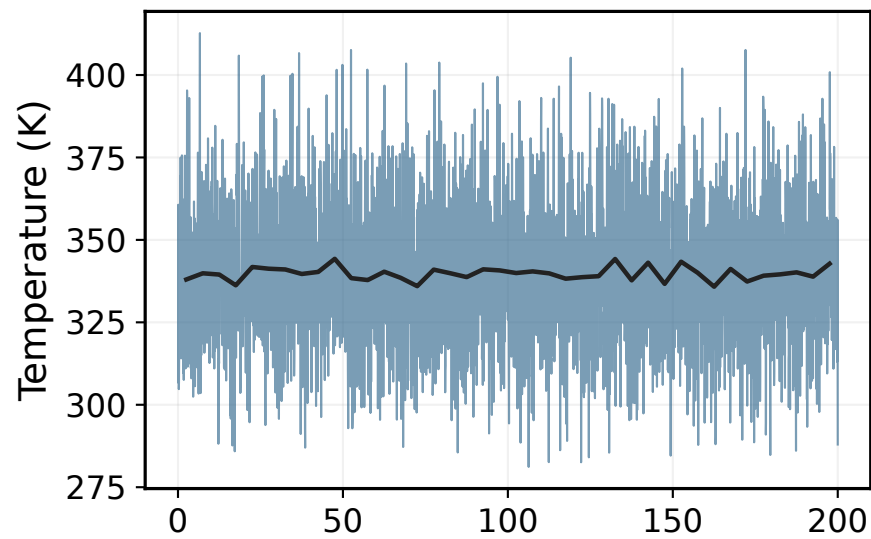
LZOC — 340 K
