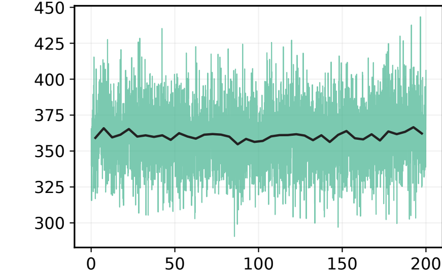
LZOC — 360 K
