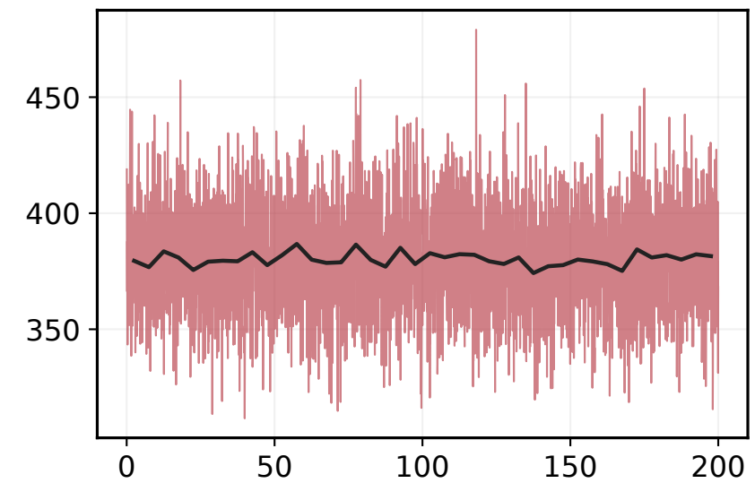
LZOC — 380 K
