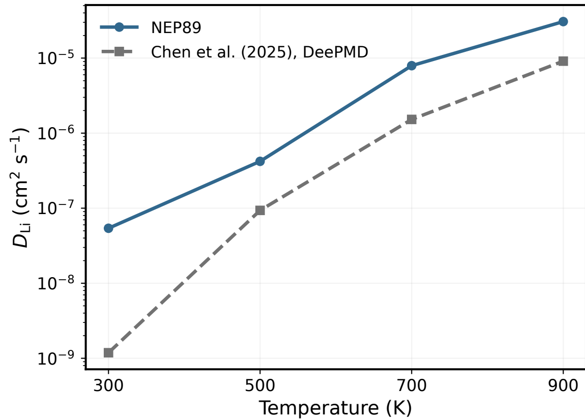
a Li-ion self-diffusion
