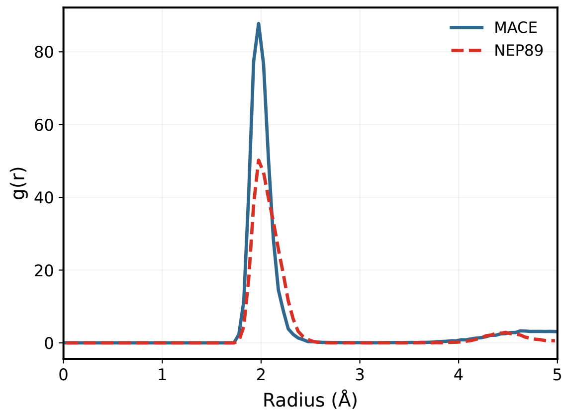
900 K: Zr-O
