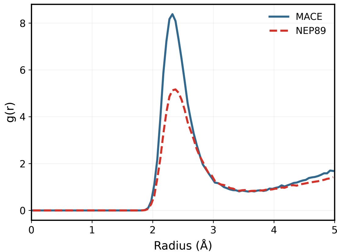
900 K: Zr-Cl
