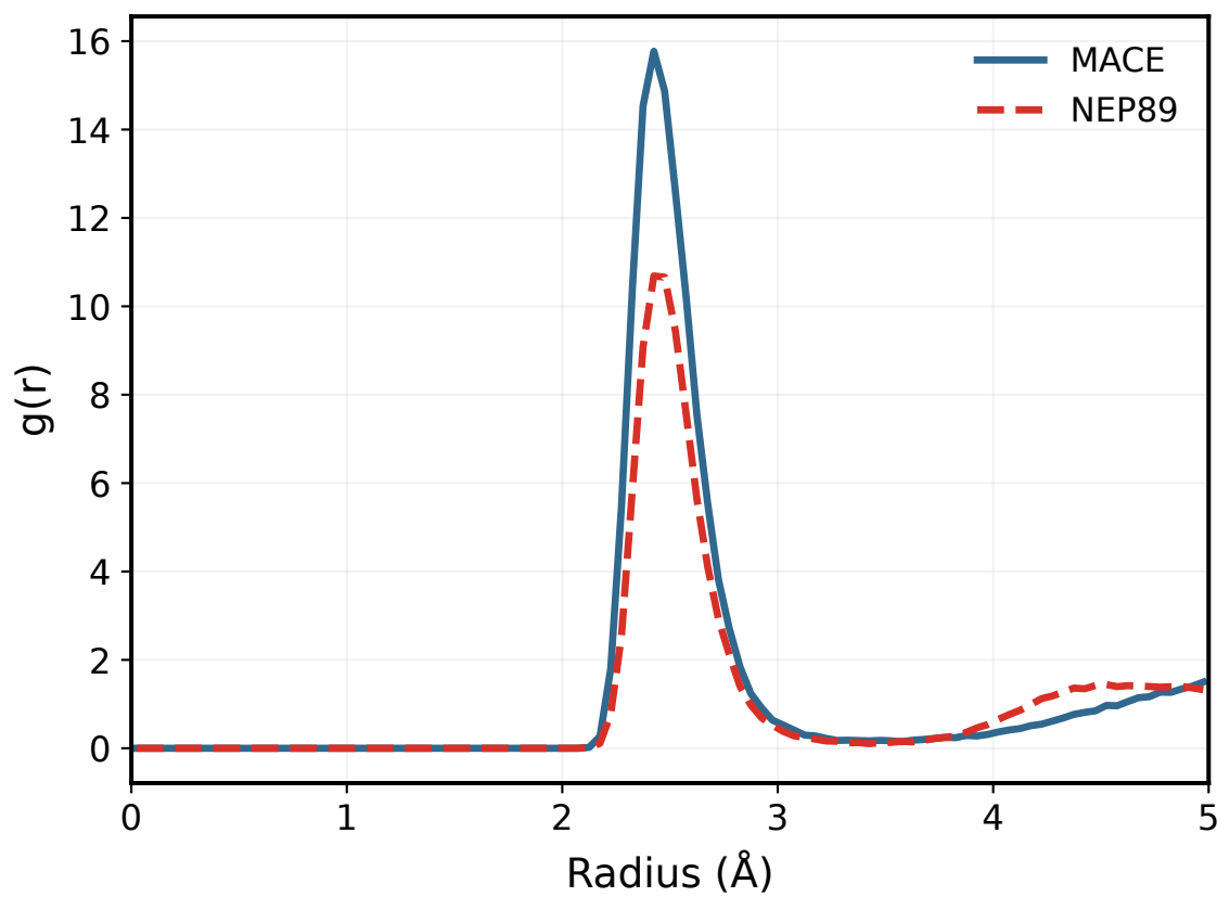
900 K: Zr-Cl
