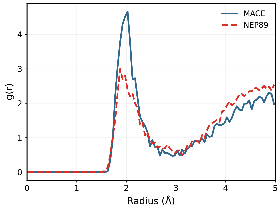
900 K: Zr-O
