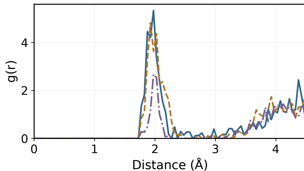
Li-O
