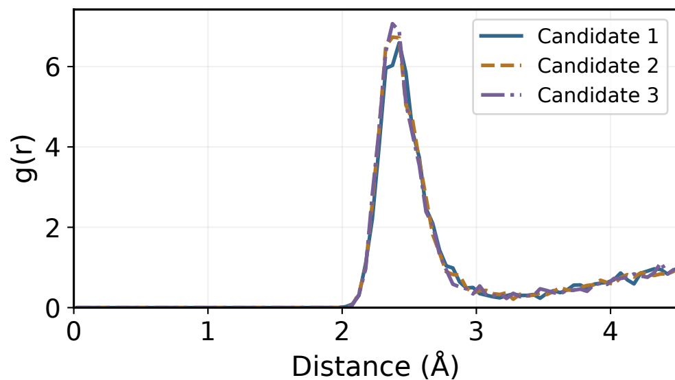
Li-Cl
