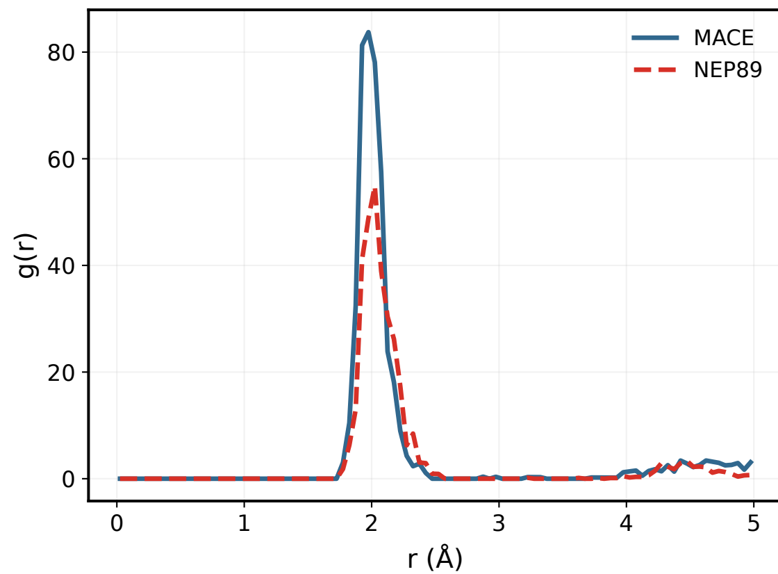
900 K: Zr-O
