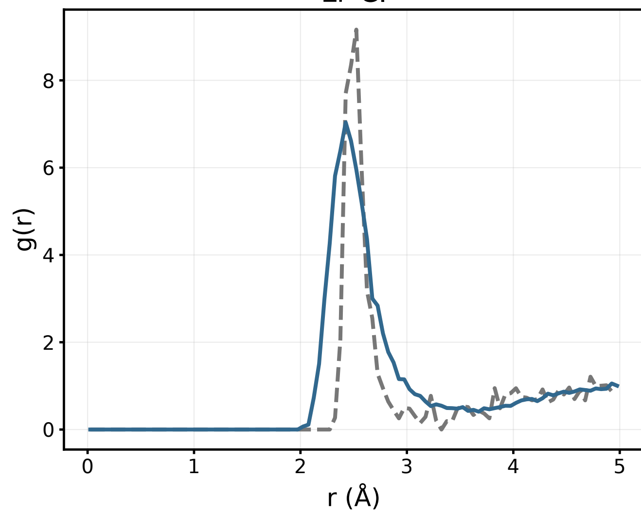
Li-Cl
