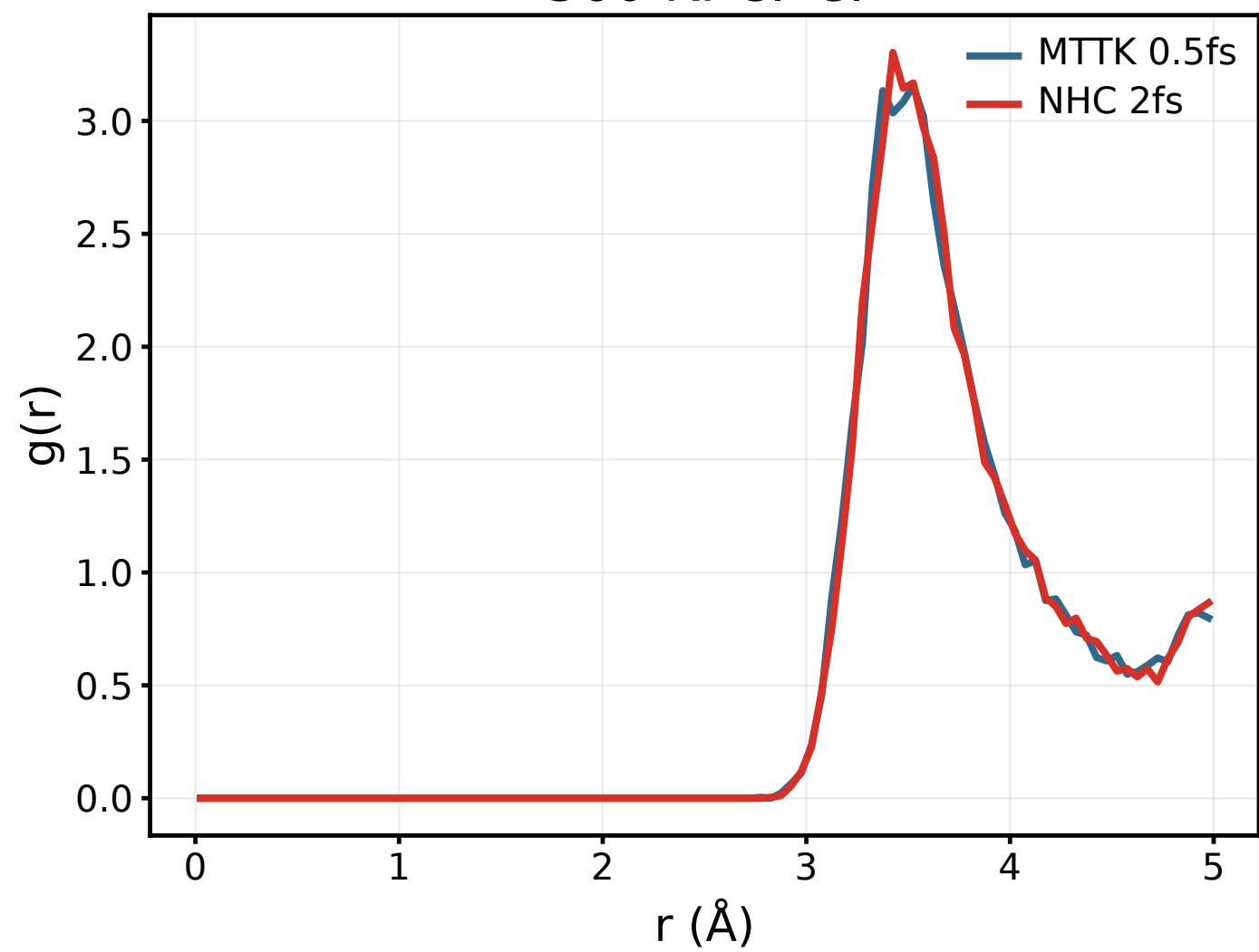
360 K: Cl-Cl
