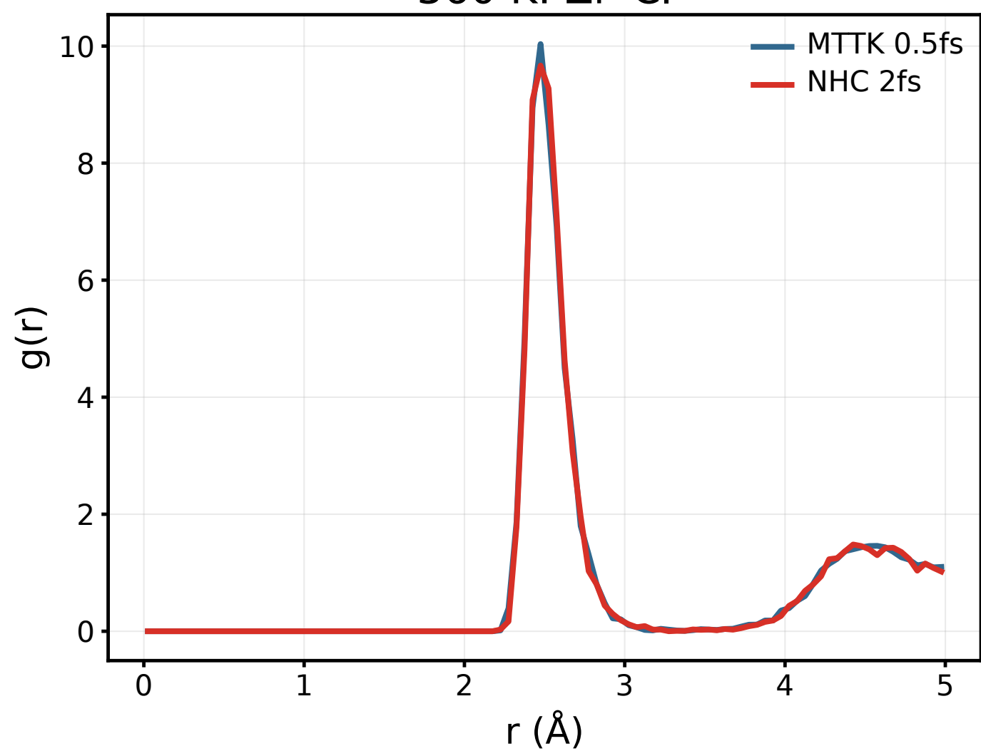
360 K: Cl-Cl
