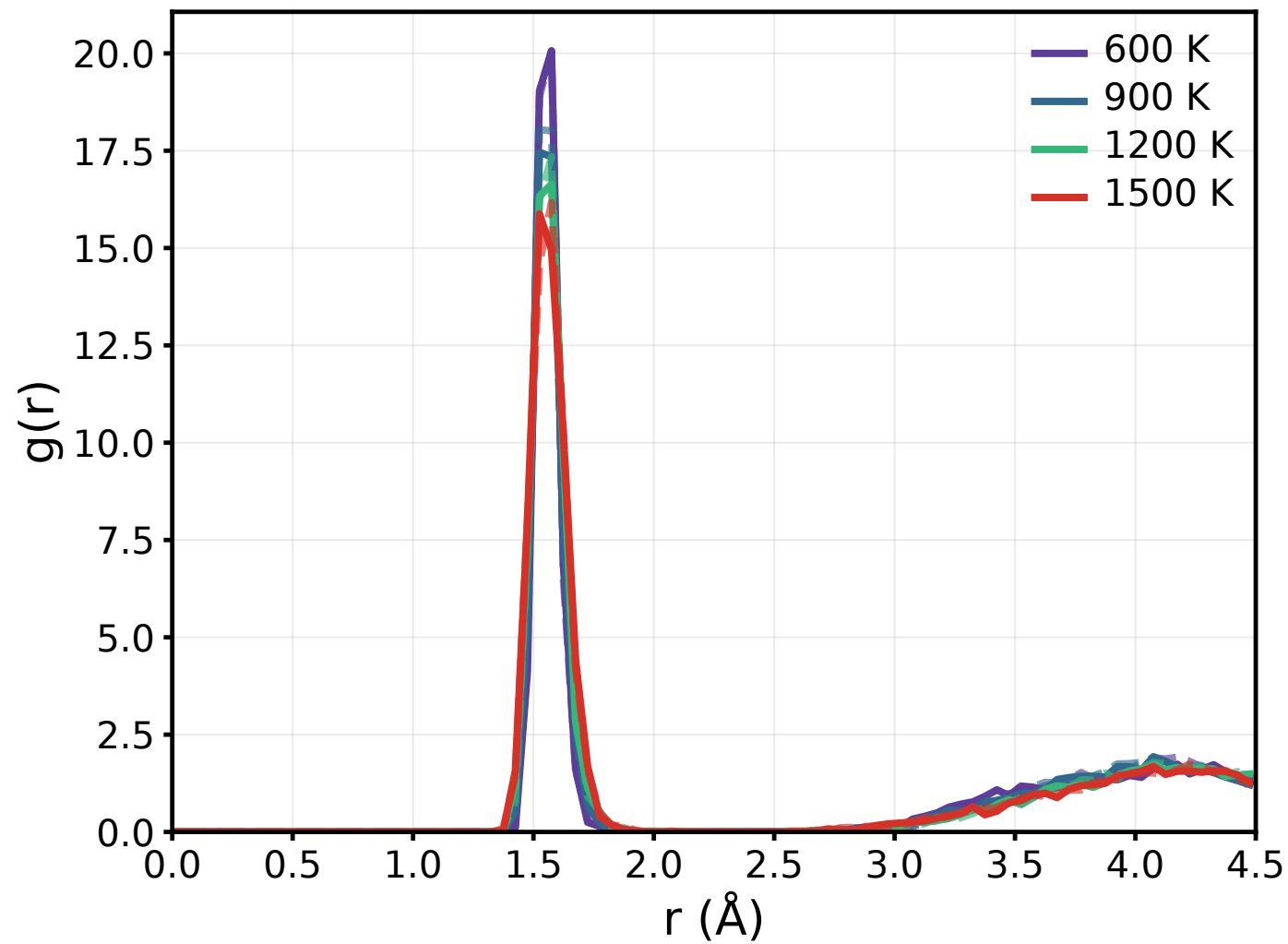
Li-O
