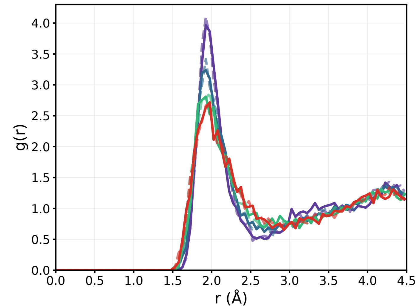
Li-O
