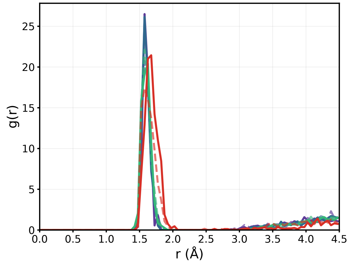
Li-N
