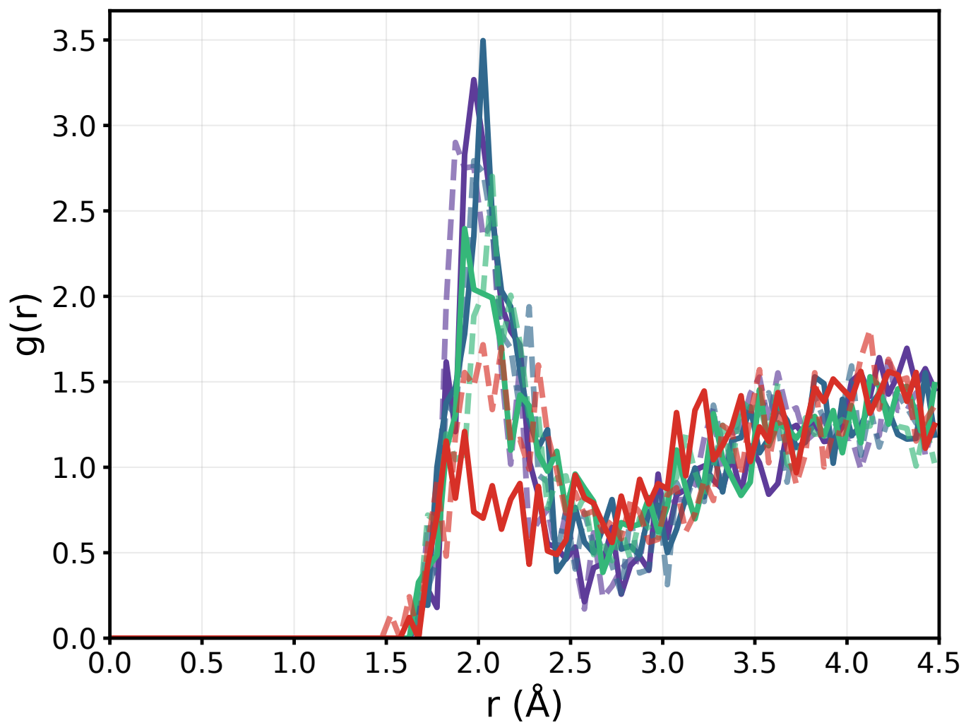
Li-N
