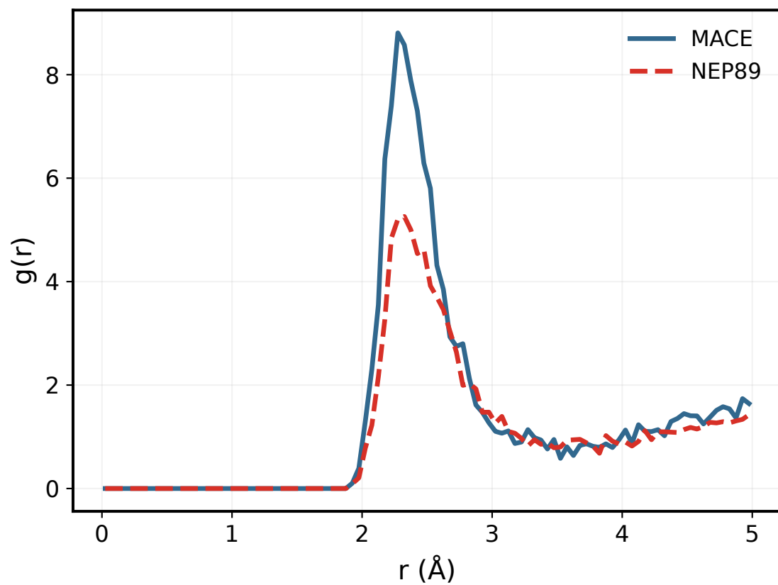
900 K: Zr-Cl
