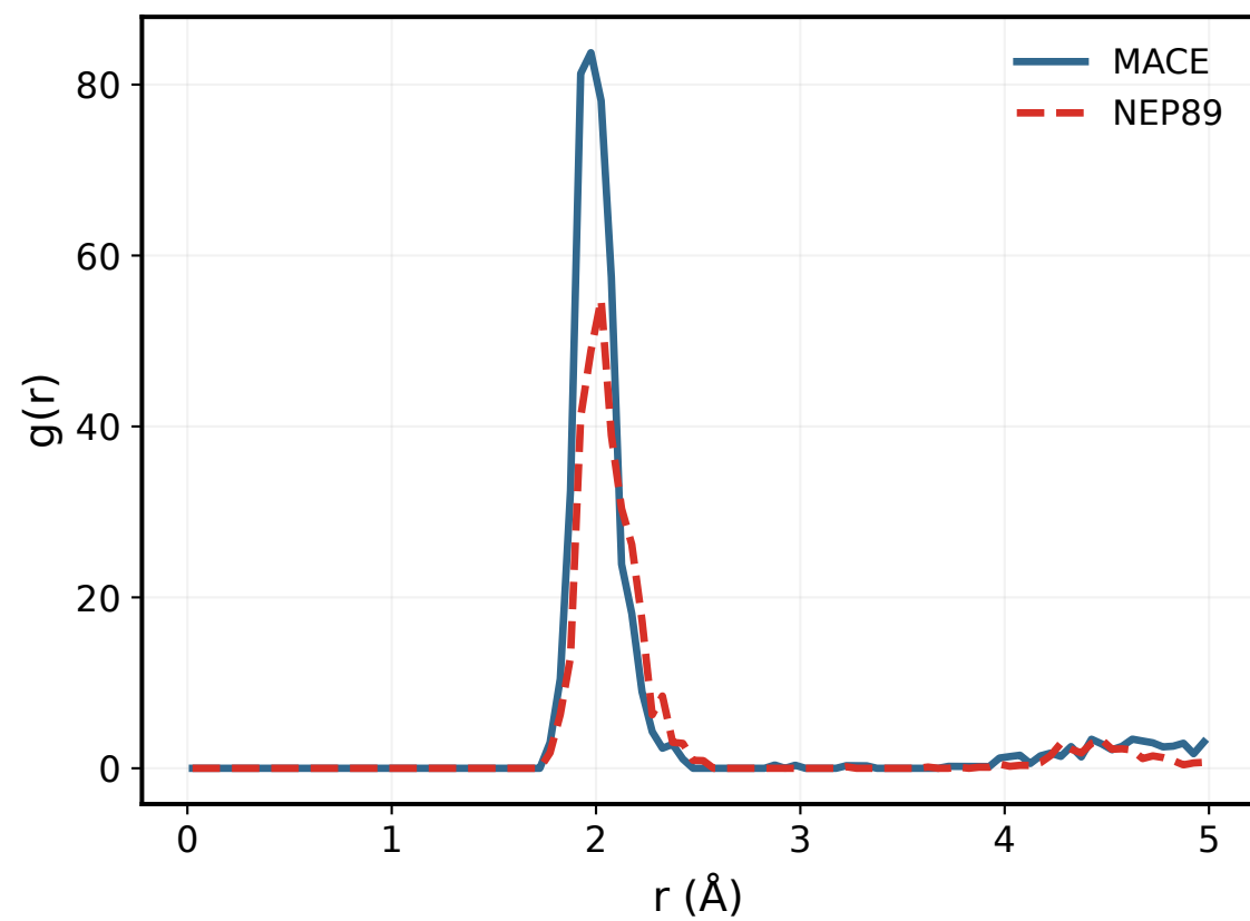
900 K: Zr-O
