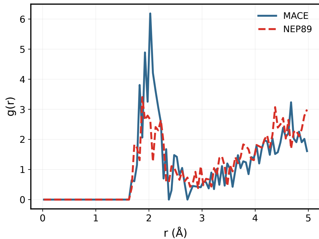
900 K: Zr-O
