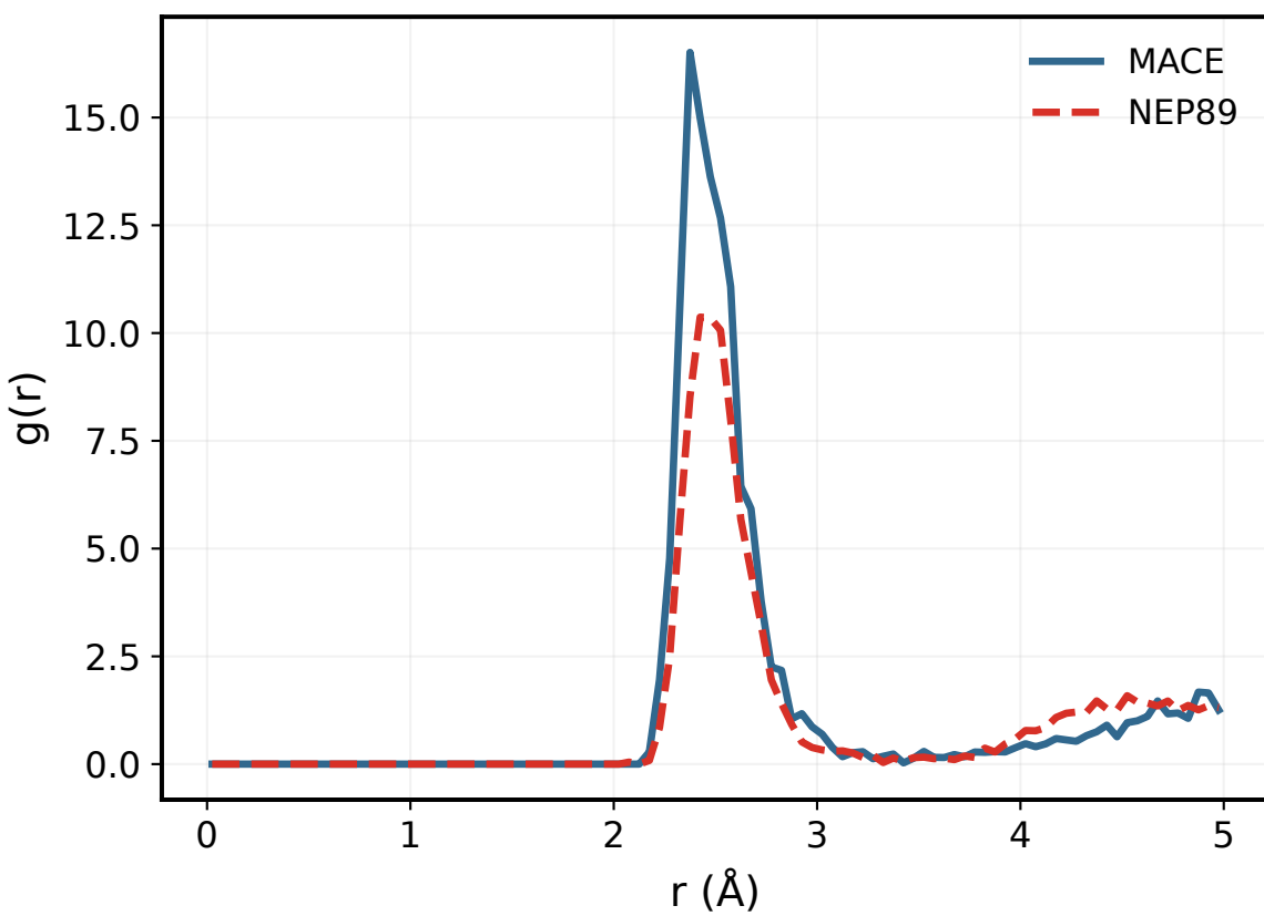
900 K: Zr-Cl
