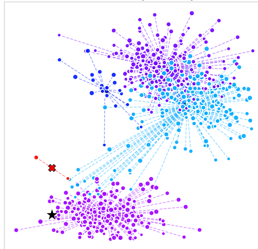
X-n716-k35 (Size 715)
