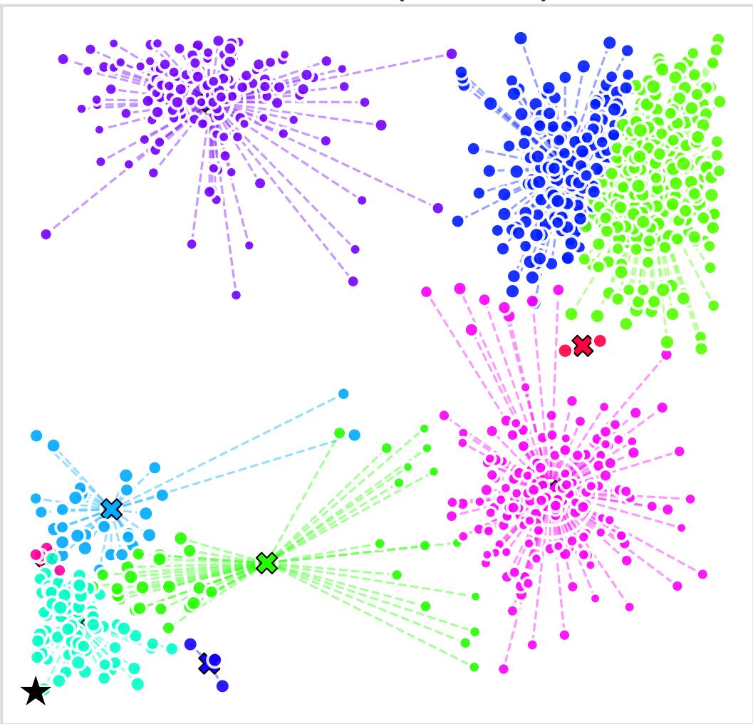
X-n979-k58 (Size 978)
