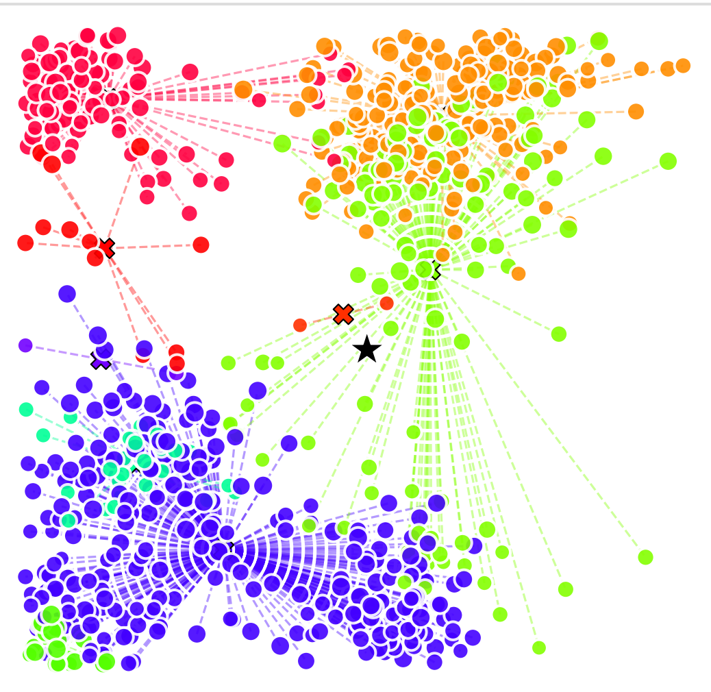
X-n819-k171 (Size 818)
