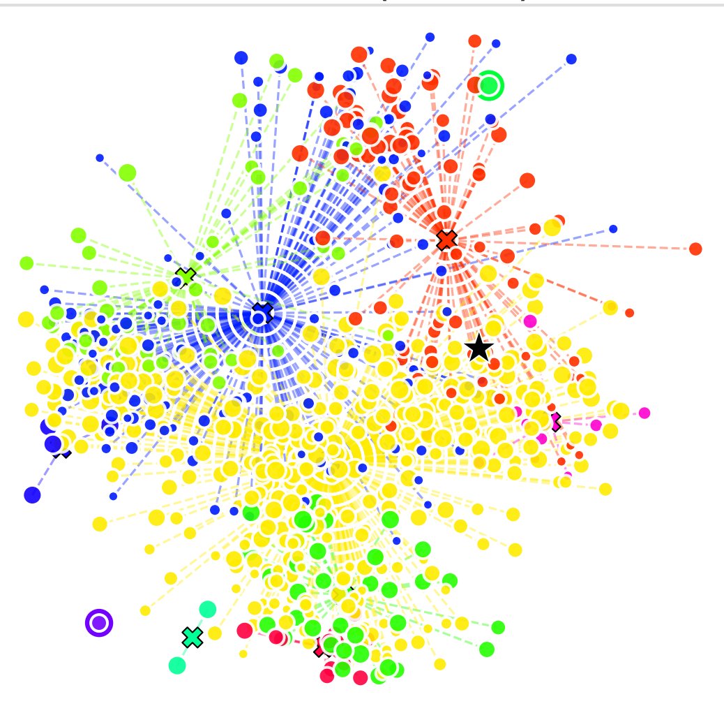
X-n749-k98 (Size 748)
