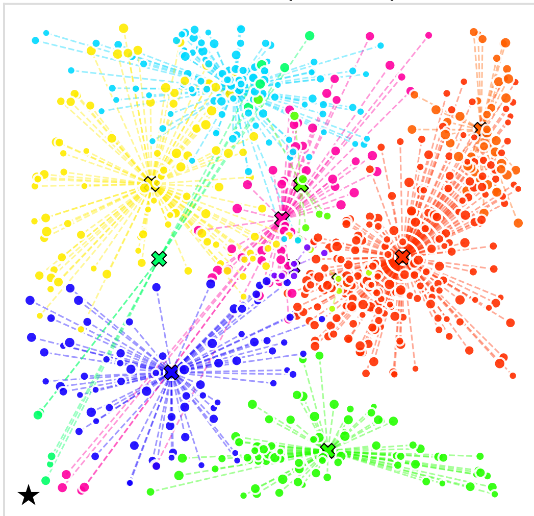
X-n701-k44 (Size 700)
