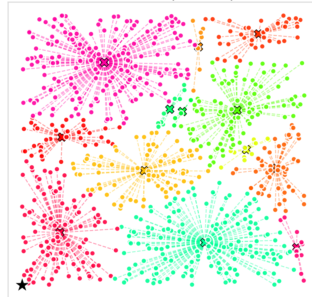
X-n801-k40 (Size 800)
