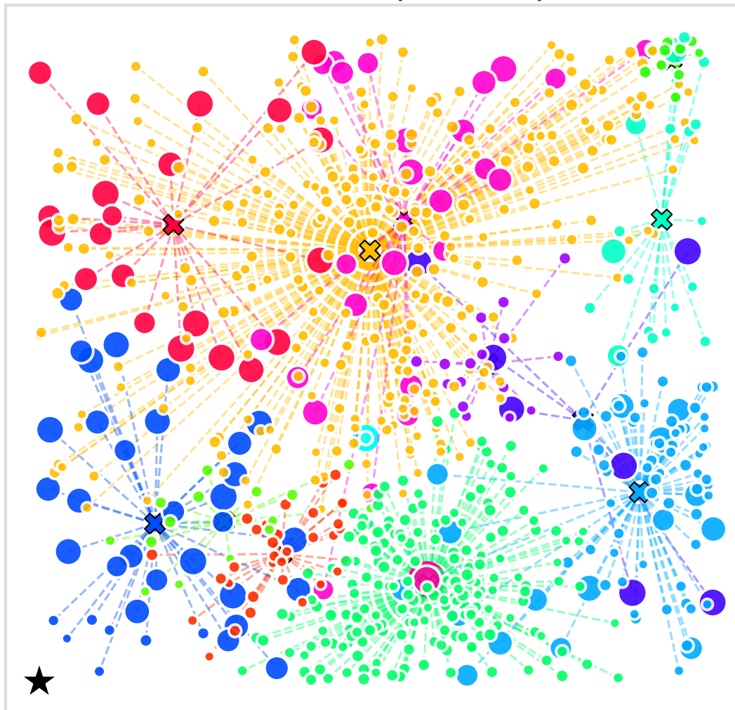
X-n766-k71 (Size 765)
