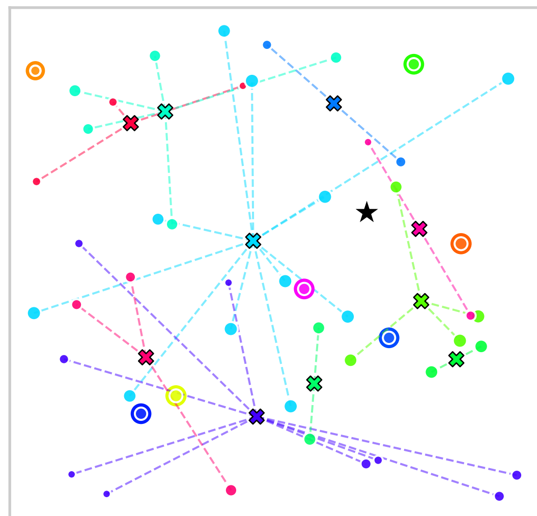
VRPL
