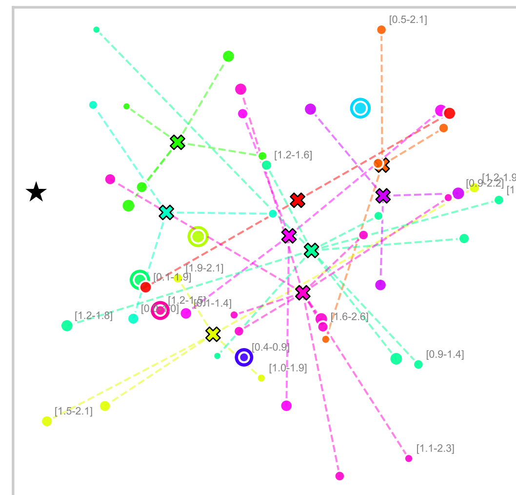
OVRPTW
