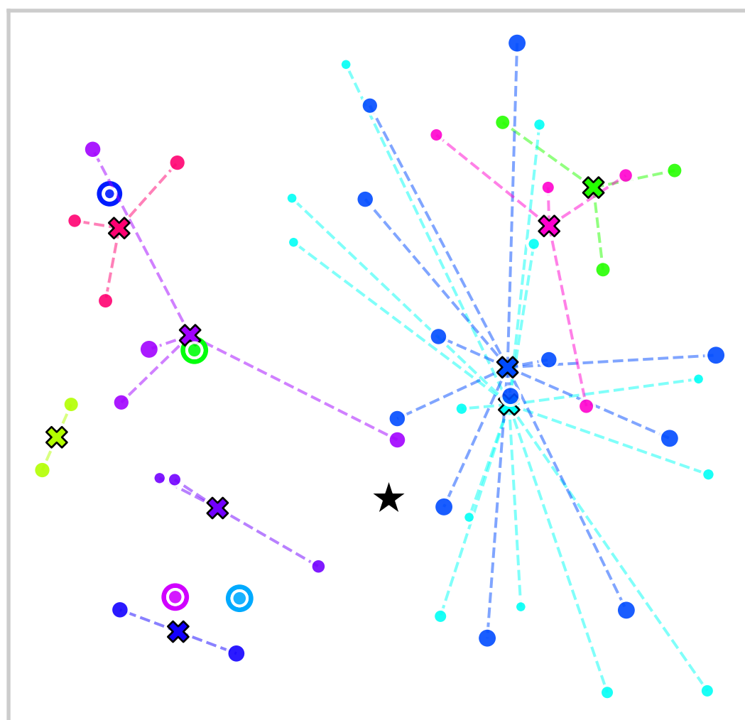
OVRPL
