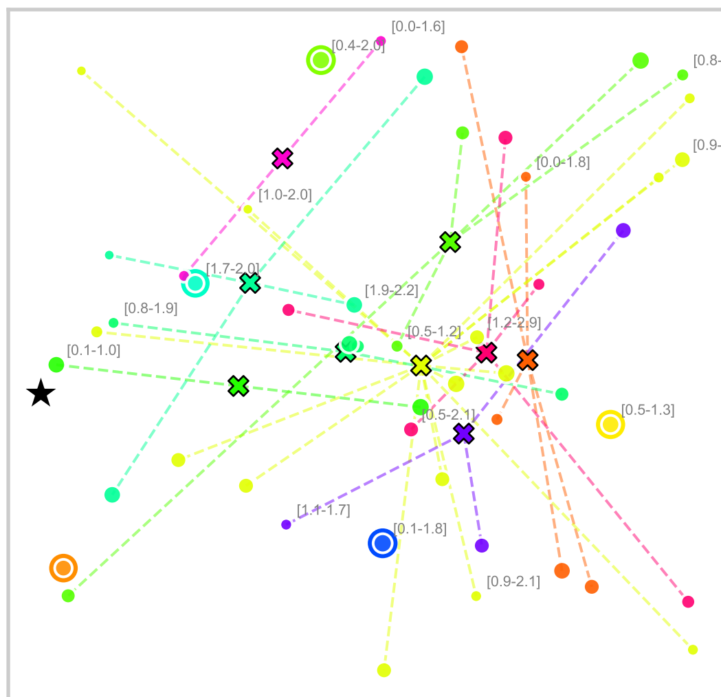
OVRPBTW
