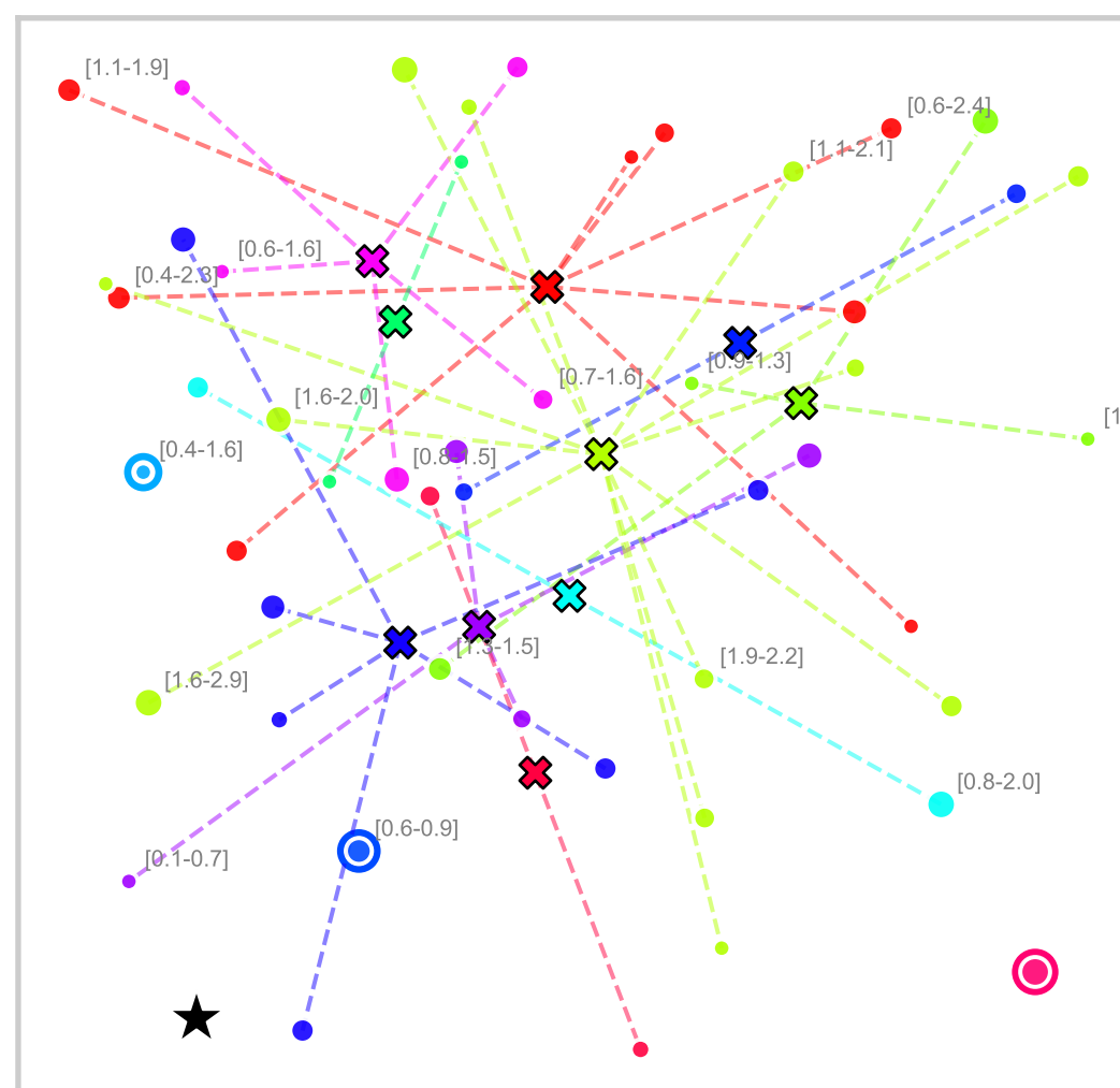
VRPBLTW
