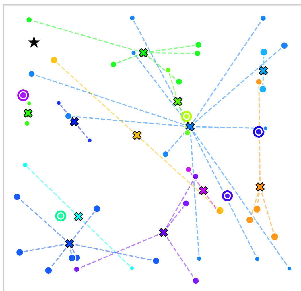
OVRPBL
