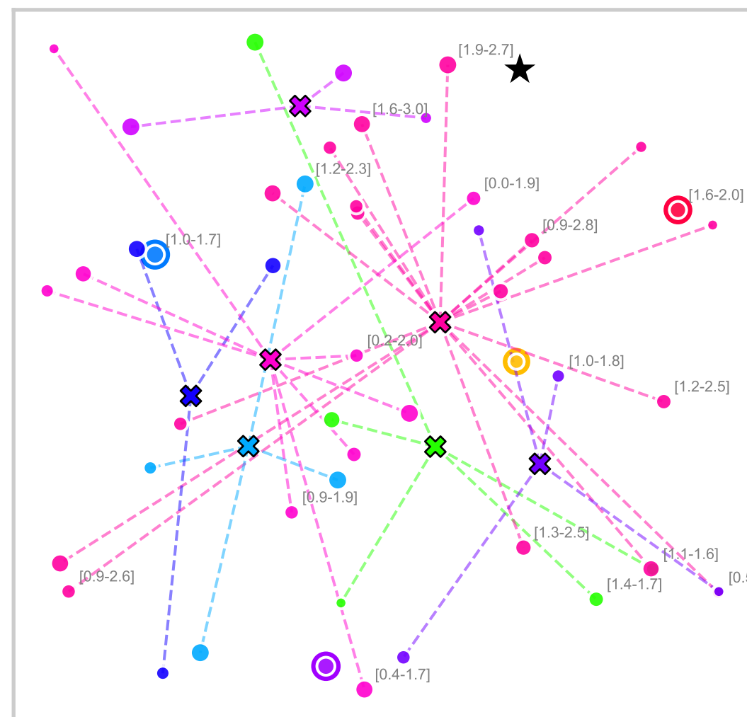
VRPBTW
