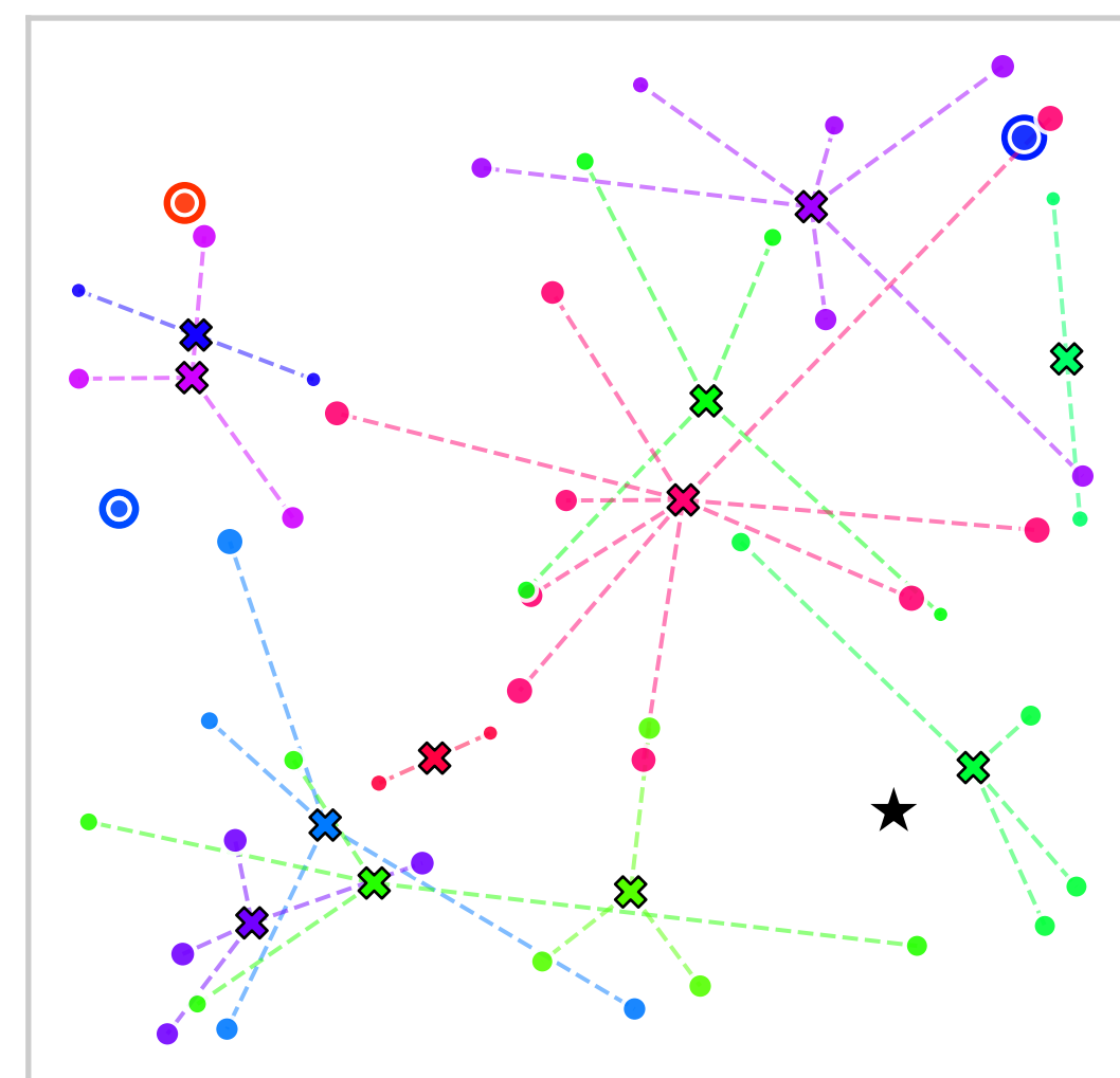
OVRPB
