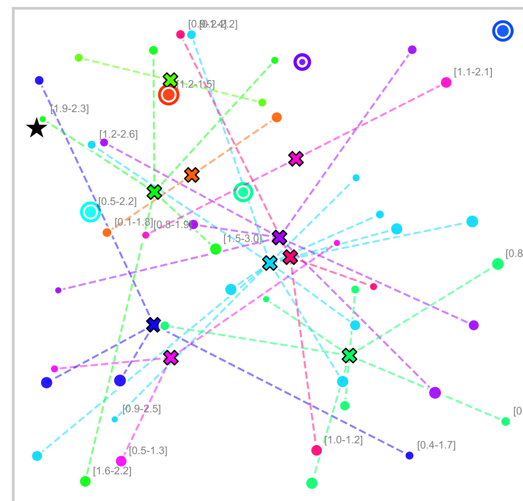
OVRPBLTW
