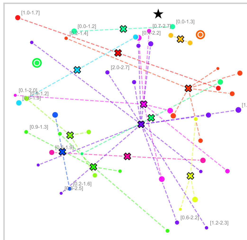
VRPLTW
