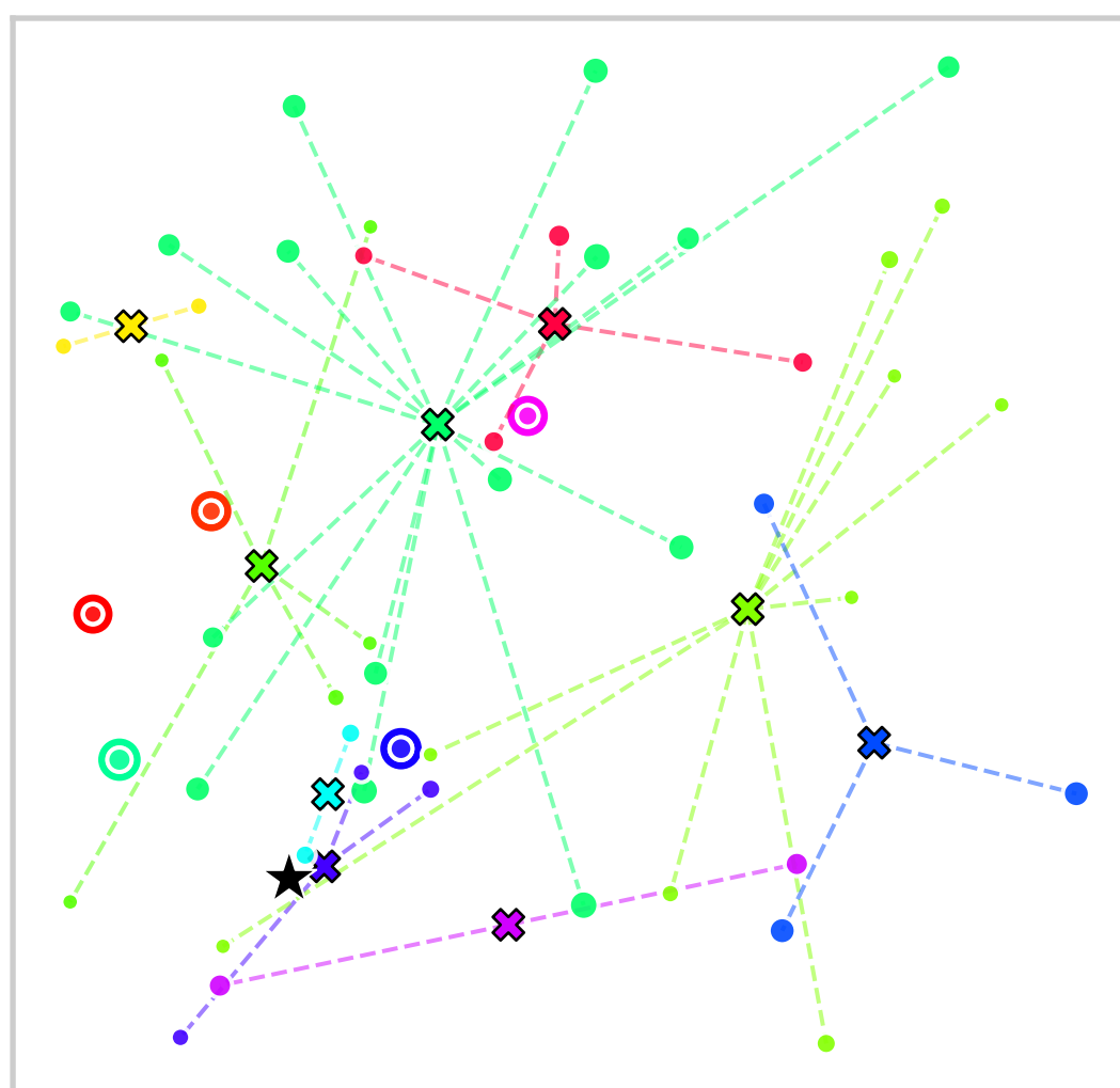
OVRP
