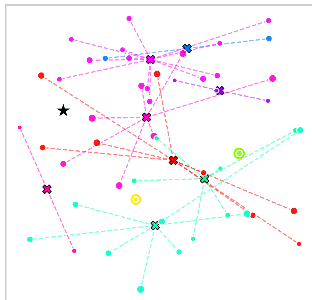
VRPBL
