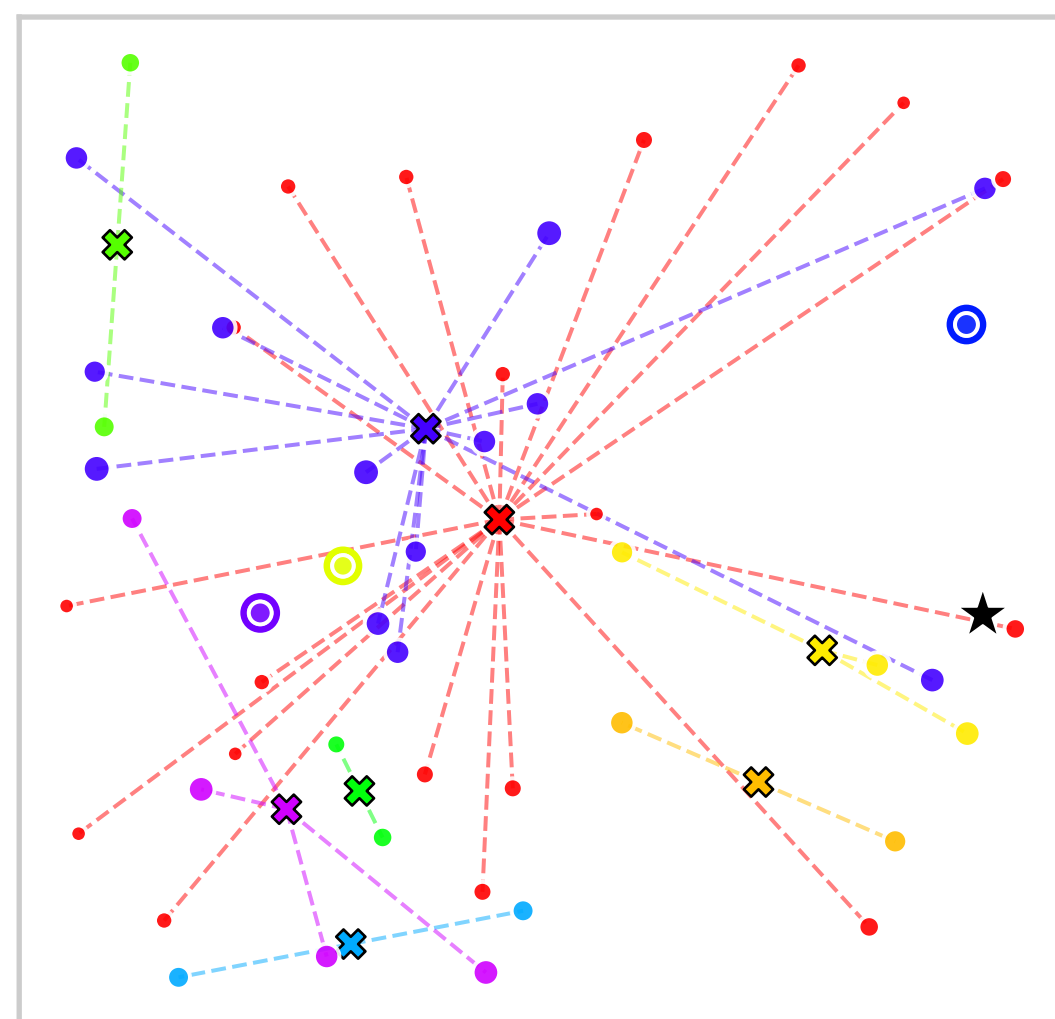
CVRP
