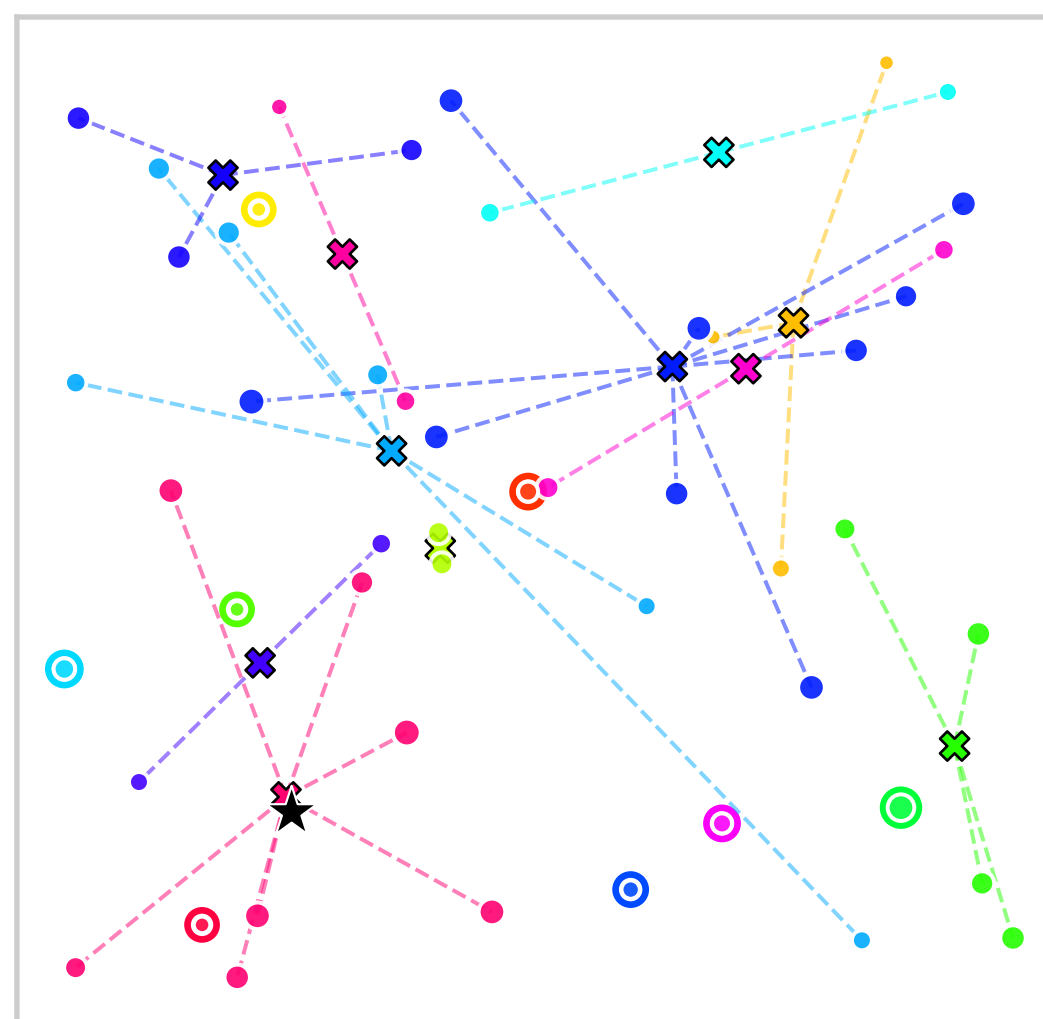
VRPB
