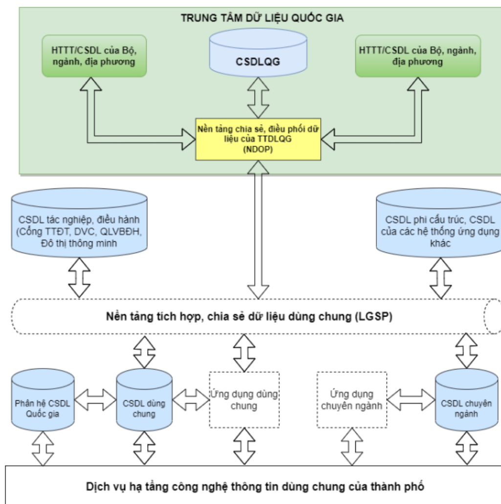
Hình 2.1 : Mô hình dữ liệu từ của Khung kiến trúc thành phố Huế 2025
