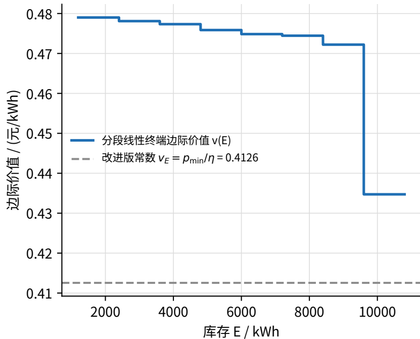
L2 终端库存价值：常数 \rightarrow 分段线性
