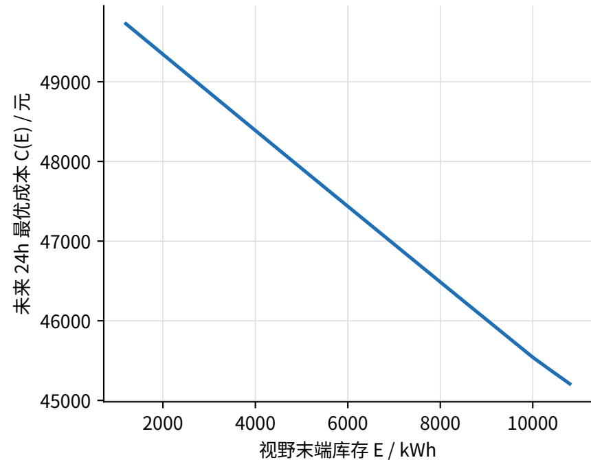
一次 Bellman 回代得到的成本函数（凸）
