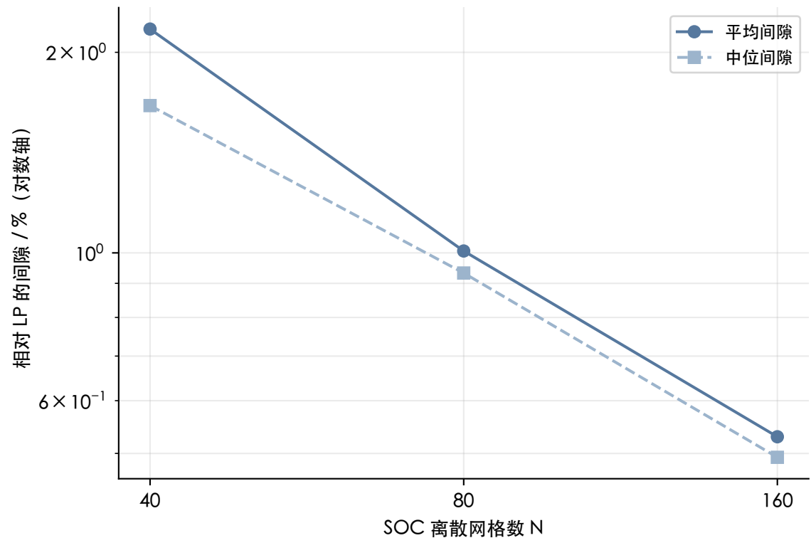
(b) DP 的离散化误差随网格加密而收敛 (约 O(1/N) )
