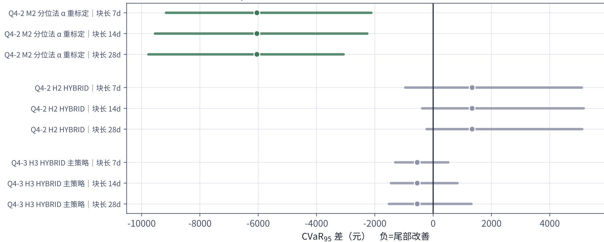
图 配对移动块 bootstrap (4000 次重采样) : 灰色表示 95% 区间跨零, 不能宣称改善
