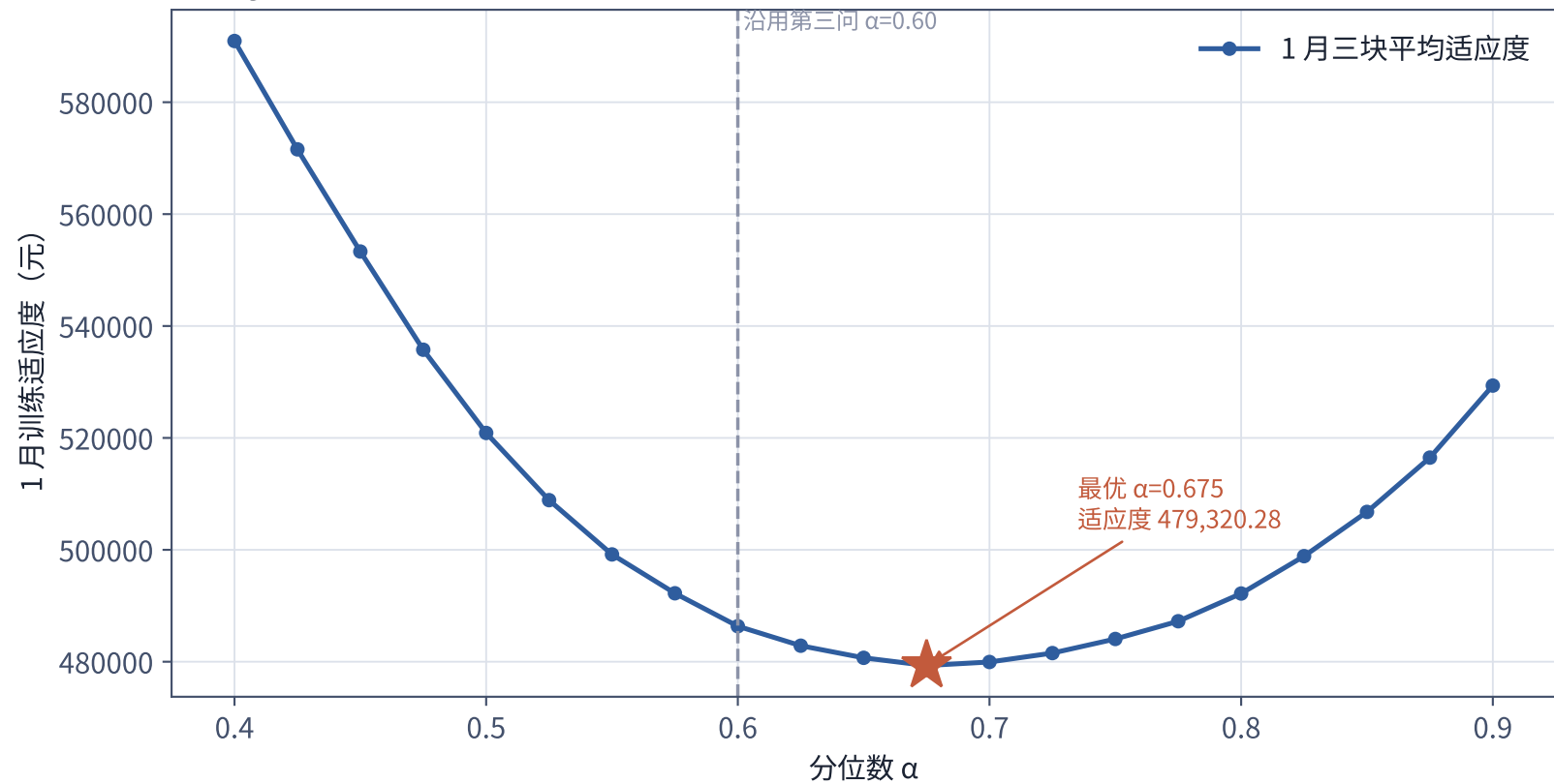
图 Q4-2 分位法一维标定：单峰、内部最优，过拟合风险最低的一次标定
