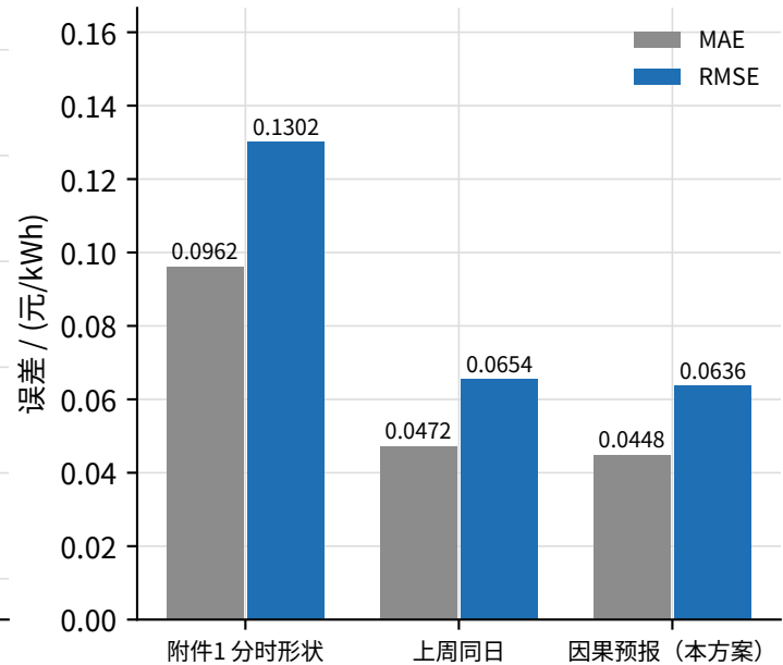
价格预报精度（越低越好）
