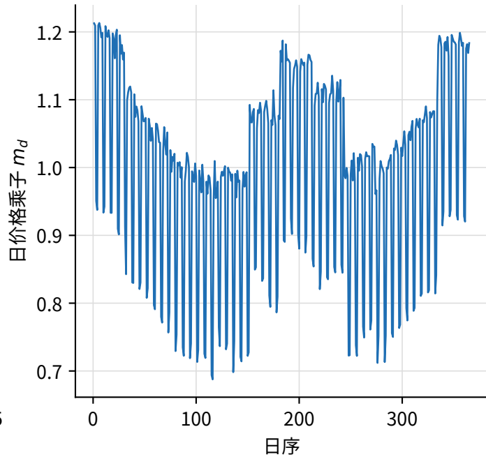
价格水平的日间波动（周期性明显）
