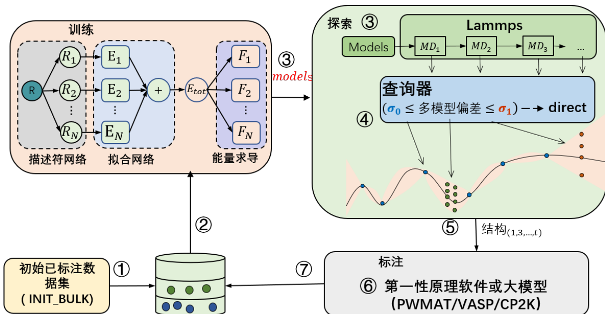
Figure 16: 主动学习流程
