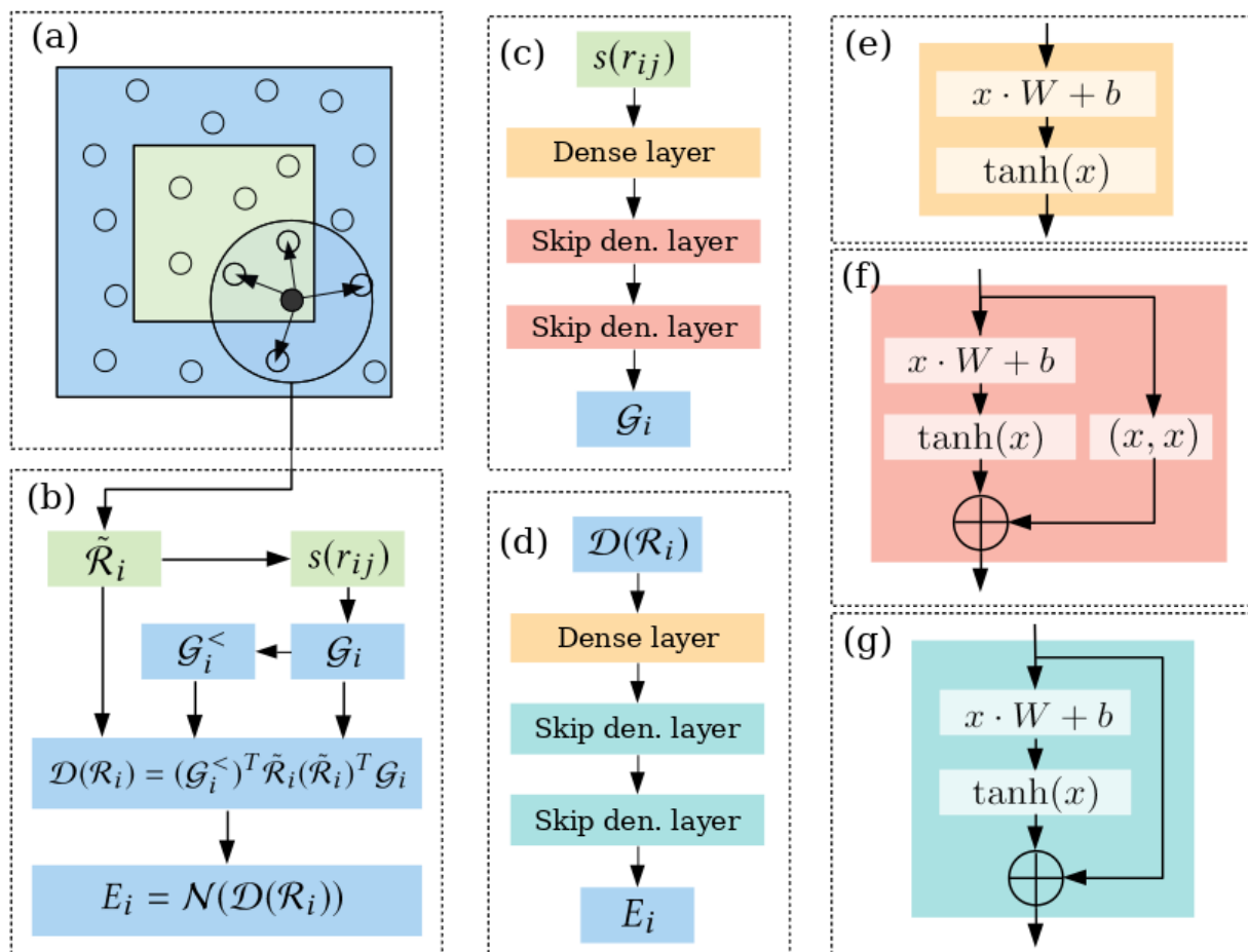
Figure 7: DP 网络结构
