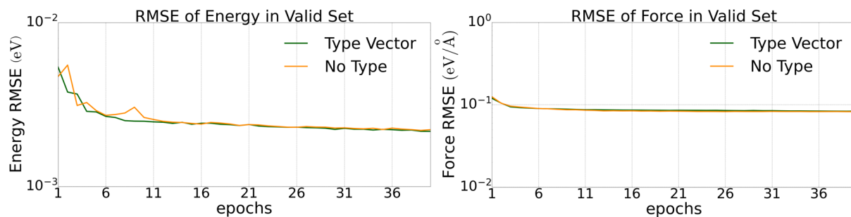
Figure 9: 四元 LiGePS 体系验证集上的能量和受力误差下降
