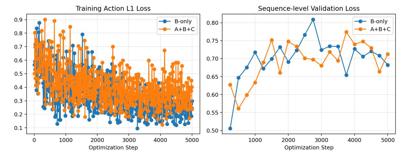
图 7: 由 SwanLab 记录指标导出的 ACT 训练 Action L1 与连续窗口验证曲线。训练损失持续下降；验证损失在早期达到最低值后出现波动，反映了小规模训练窗口上的过拟合。
