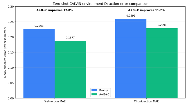
图 8: 环境 D 上的 zero-shot 动作误差。与 B-only 相比，A+B+C 联合训练使 first-action MAE 下降 17.0%，chunk-action MAE 下降 11.7%。
